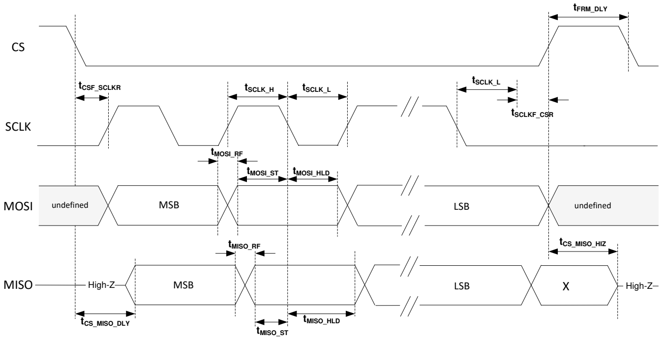
图 6-1. SPI 时序图
