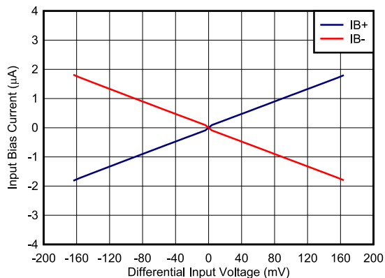
图 6-14. 输入偏置电流与差分输入电压间的关系
