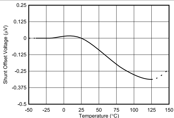
图 6-4. 分流输入失调电压与温度间的关系
