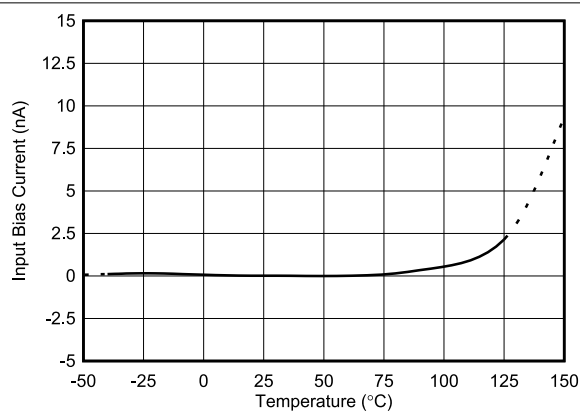
图 6-16. 输入偏置电流与温度间的关系
