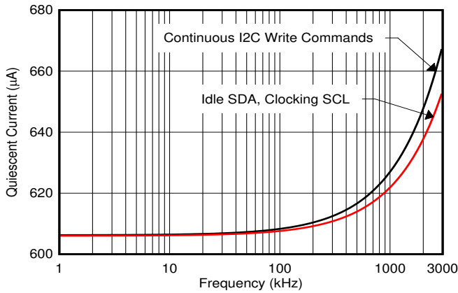
图 6-22. 工作 I_Q 与时钟频率间的关系
