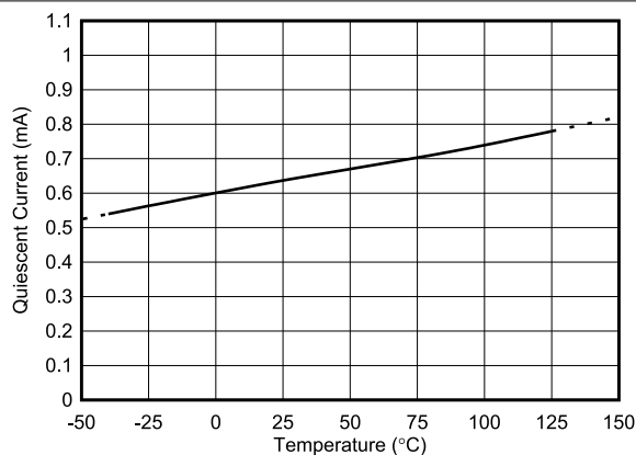
图 6-18. 工作 I_Q 与温度间的关系
