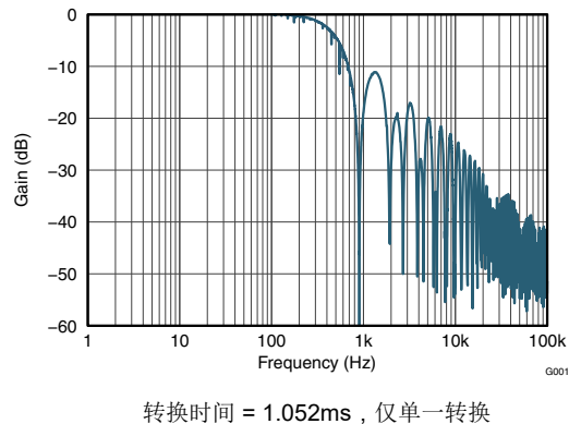
图 7-3. ADC 频率响应
