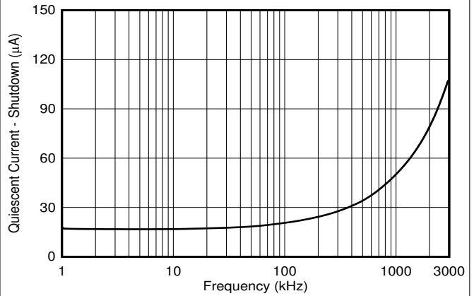
图 6-23. 关断 I_Q 与时钟频率间的关系
