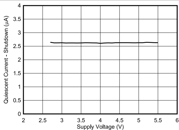
图 6-20. 关断 I_Q 与电源电压间的关系
