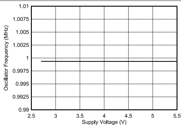
图 6-24. 内部时钟频率与电源间的关系
