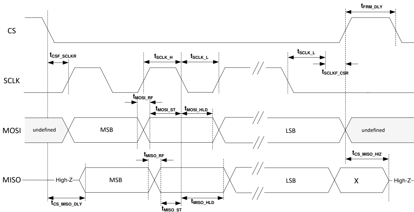
图 6-1. SPI 时序图
