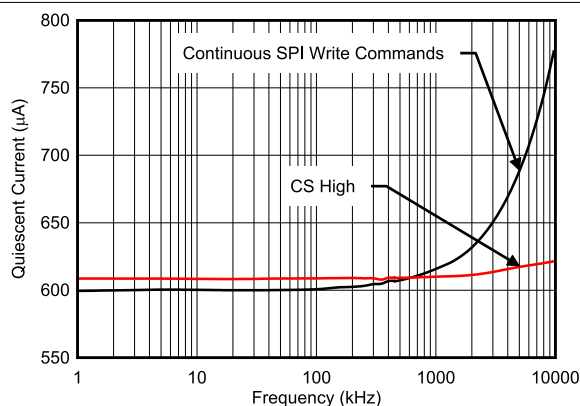
图 6-22. 工作 I_Q 与时钟频率间的关系
