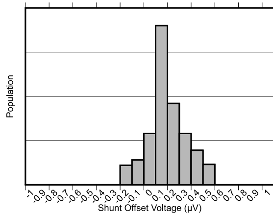
图 6-3. 分流输入失调电压产生分布图
