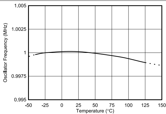
图 6-25. 内部时钟频率与温度间的关系
