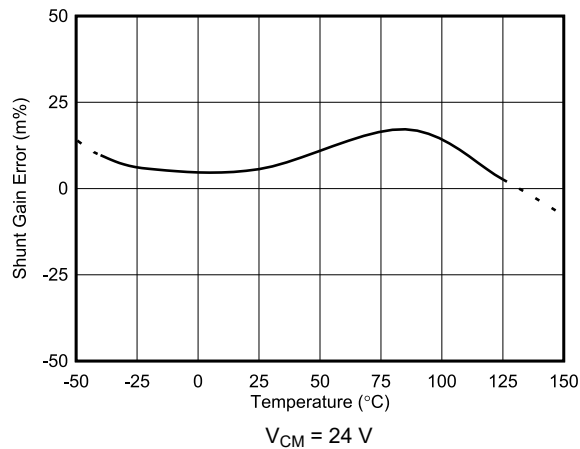
图 6-8. 分流输入增益误差与温度间的关系
