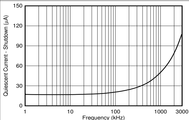
图 6-23. 关断 I_Q 与时钟频率间的关系
