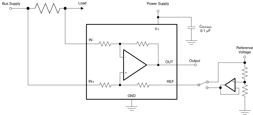
图 7-3. 双向应用原理图
