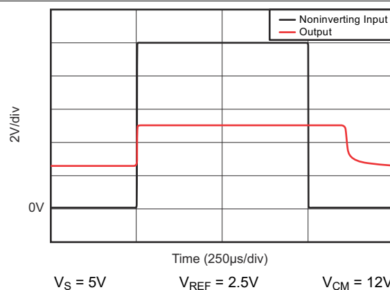
图 5-20. 同相差分输入过载
