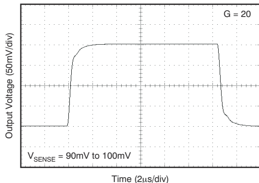
图 6-14. Step Response
