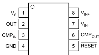
图 5-1. DGK 封装 8 引脚 VSSOP 顶视图
