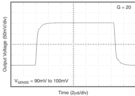
图 6-13. 阶跃响应
