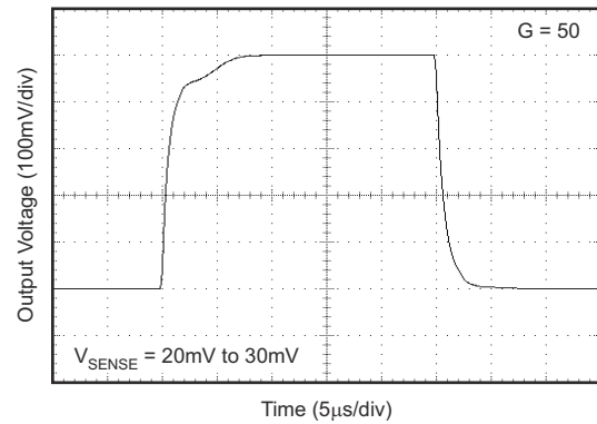
图 6-14. 阶跃响应
