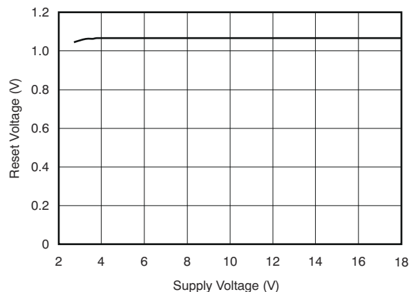
图 6-22. 比较器复位电压与电源电压关系图
