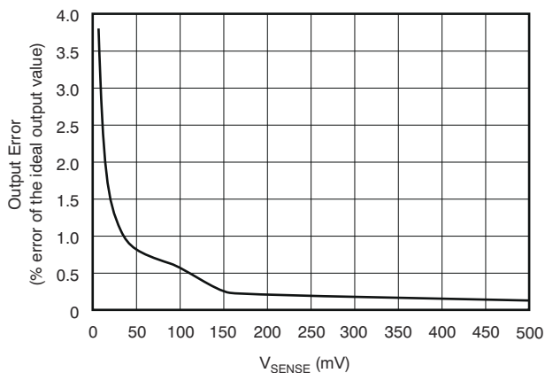
图 6-5. 增益误差与 V_{SENSE} )
