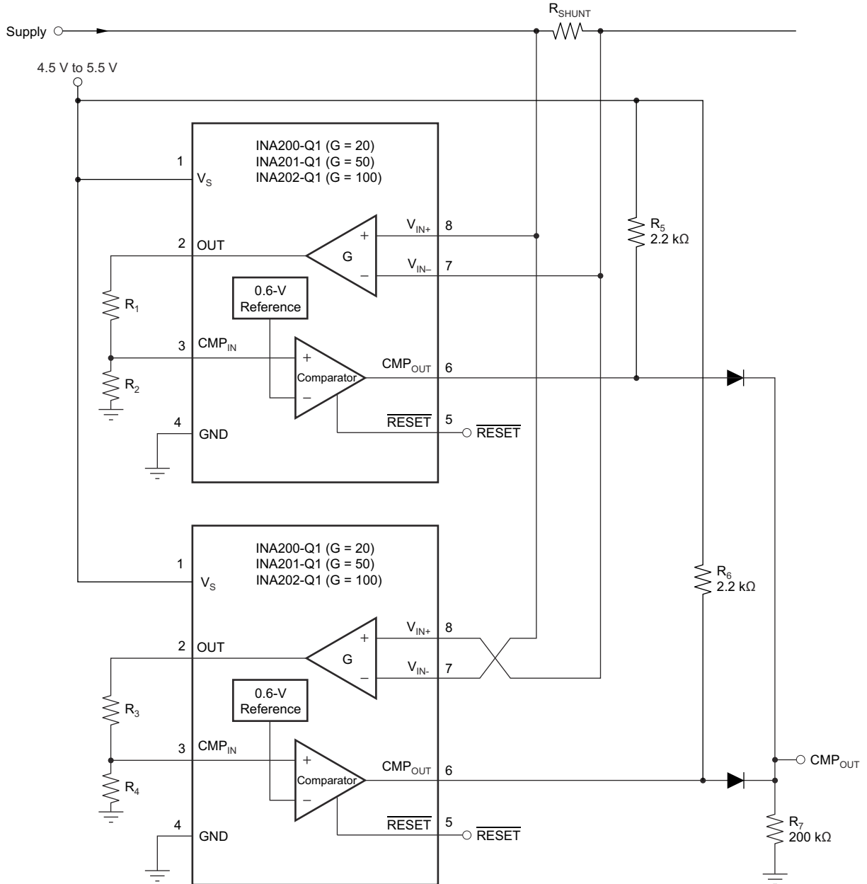
图 9-8. 双向过流比较器
