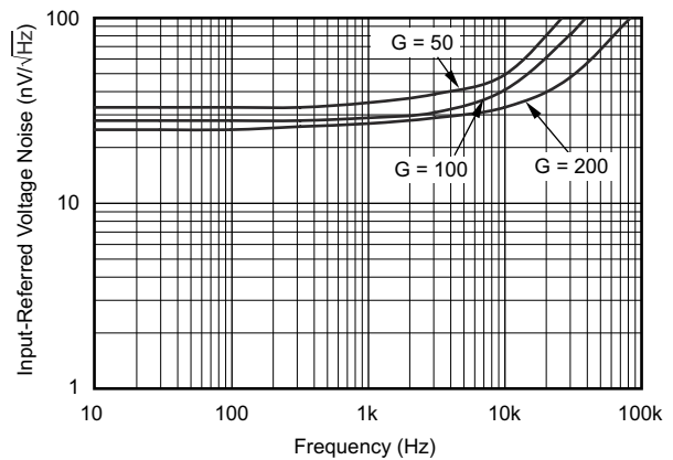
图 7-12. 输入基准电压噪声与频率间的关系
