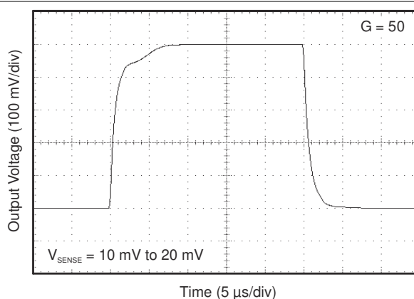
图 6-16. Step Response
