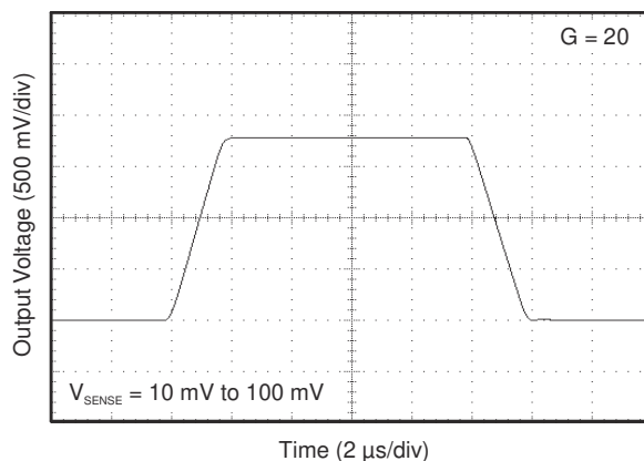
图 6-14. Step Response
