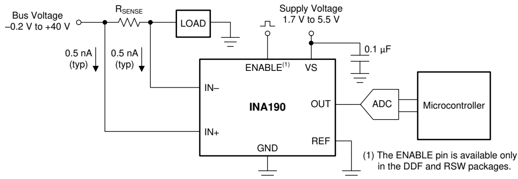
典型应用
