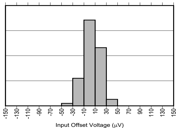
图 5-1. INA187 输入失调电压产生分布图
