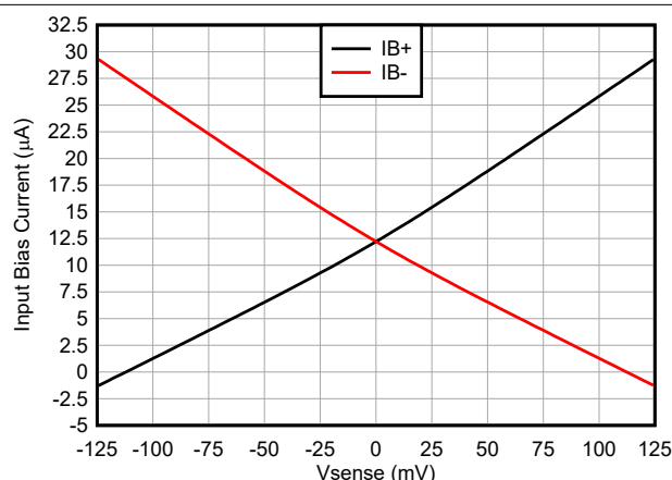
图 5-13. INA187 增益 = 20V/V，输入偏置电流与 V_{\text{SENSE}} 间的关系
