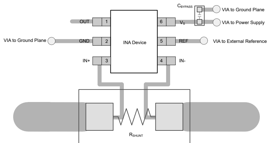
图 7-3. INA187 SOT-23 6 引脚 (DBV) 封装建议布局
