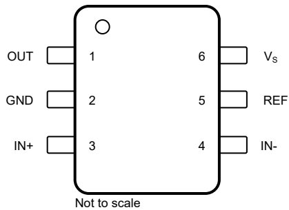
图 4-1. INA187 : DBV 封装 6 引脚 SOT-23 顶视图
