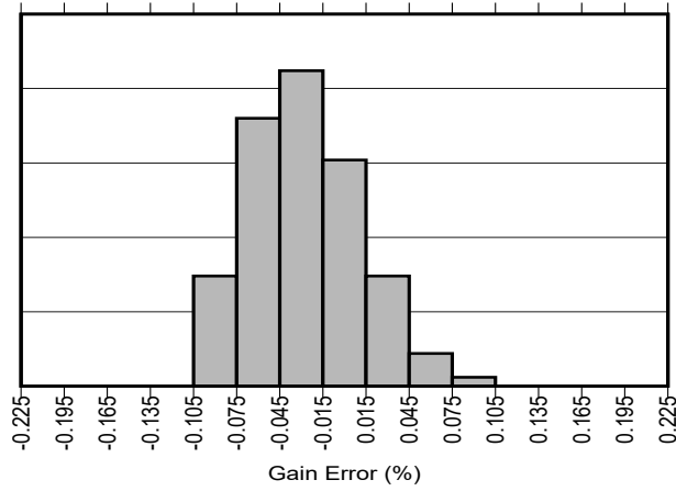
图 5-7. INA187 增益误差产生分布图
