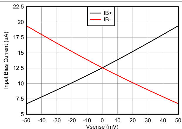
图 5-14. INA187 增益 = 50V/V，输入偏置电流与 V_{\text{SENSE}} 间的关系
