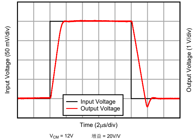
图 5-30. 大阶跃响应
