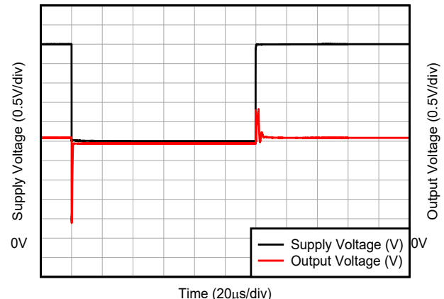
图 5-32. 欠压恢复
