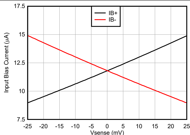
图 5-15. INA187 增益 = 100V/V，输入偏置电流与 V_{\text{SENSE}} 间的关系
