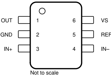
图 5-1. INA181-Q1 : DBV 封装 6 引脚 SOT-23 顶视图
