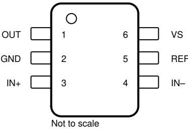
图 5-1. INA181 : DBV 封装 6 引脚 SOT-23 顶视图
