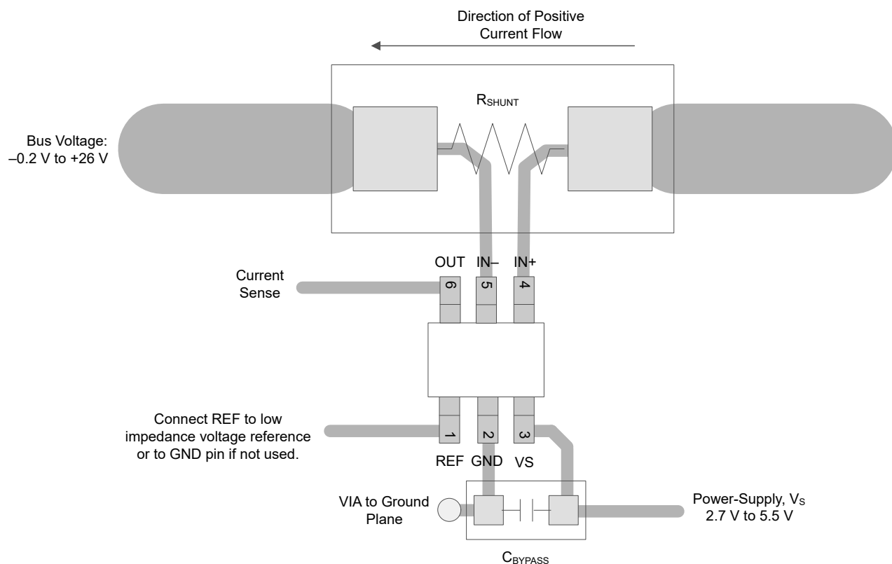
图 8-11. 单通道推荐布局 (SC70)
