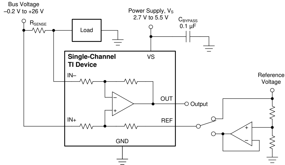
图 7-7. 双向应用
