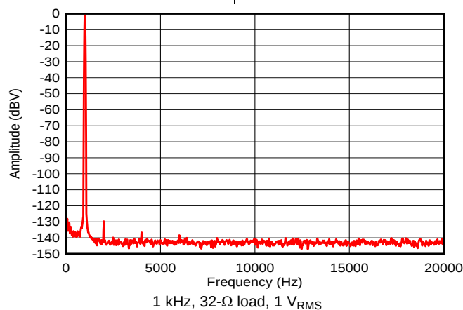
图 59. Output Spectrum
