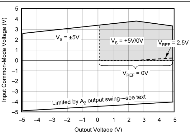
图 6-4. 输入共模范围与输出电压间的关系, V_s = \pm 5V , G = 5
