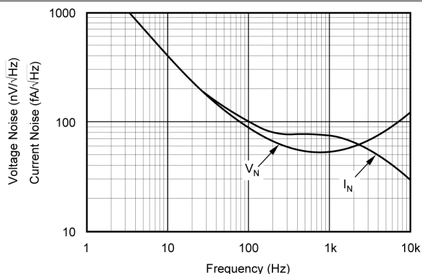
图 5-7. 电压和电流噪声密度与频率间的关系 (RTI)
