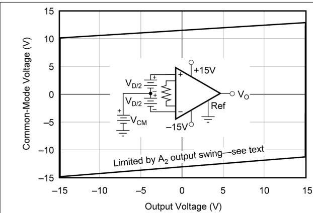
图 6-3. 输入共模范围与输出电压间的关系, V_s = \pm 15V , G = 5
