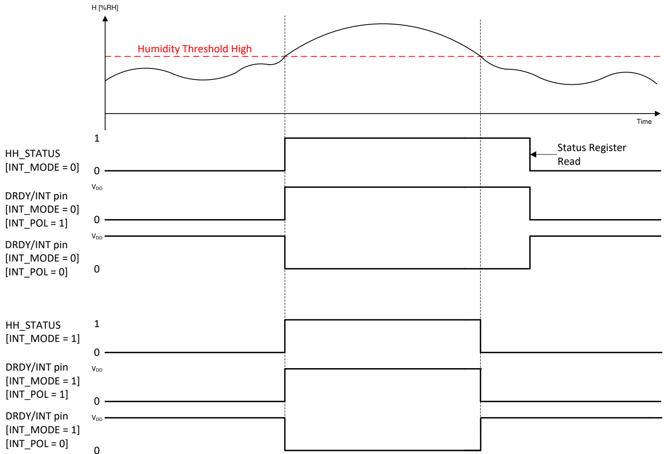
图 7-5. 阈值中断 - 湿度高
