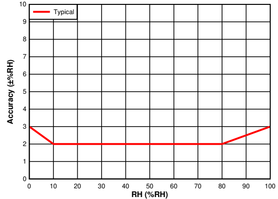
RH 精度 (TA = 30°C)
