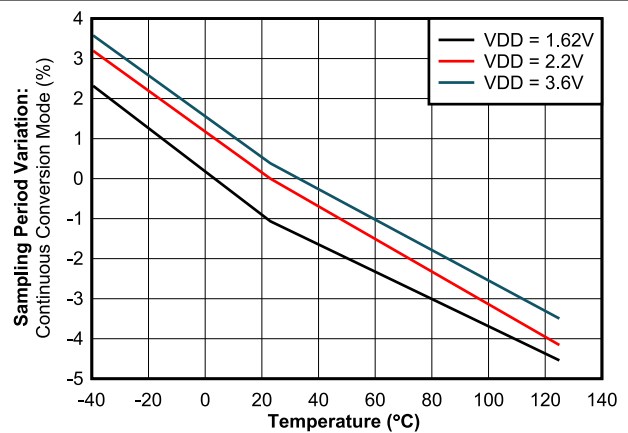
图 6-13. 采样周期变化 (连续转换模式) 与温度间的关系
