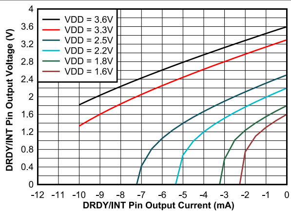
图 6-12. 输出电压 (DRDY/INT 引脚) 与输出电流 (逻辑高电平) 间的关系
