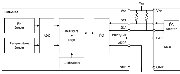
典型应用
