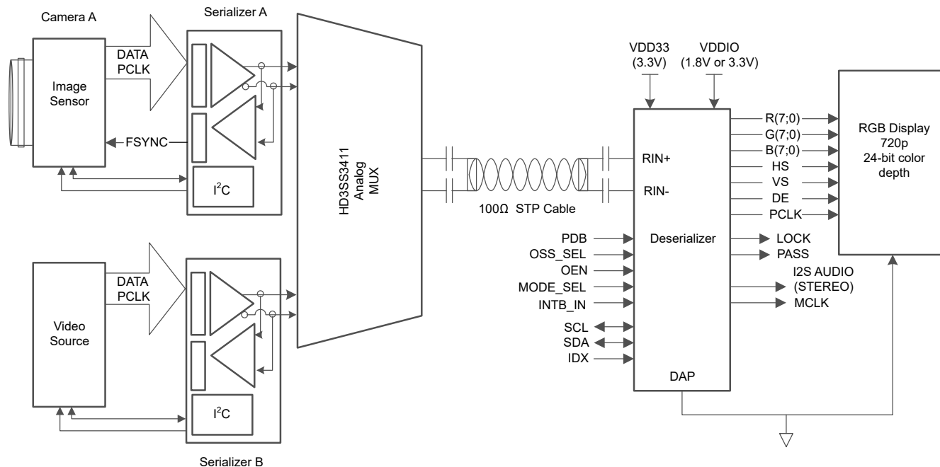
图 7-1. FPD Link III Application
