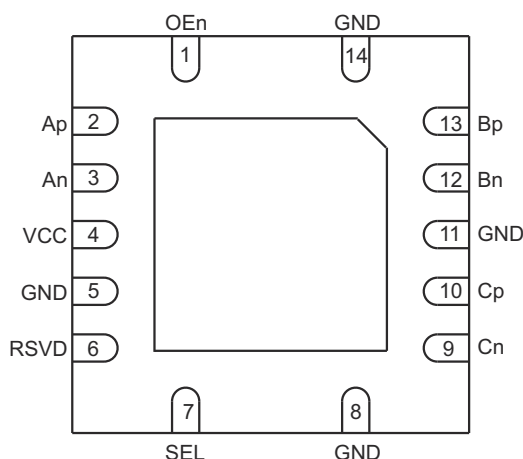
图 4-1. RWA Package, 14-Pin WQFN (Top View)
