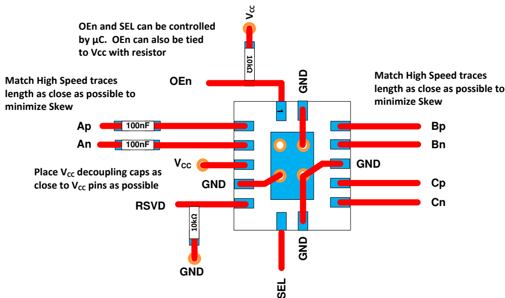
图 7-7. Layout
