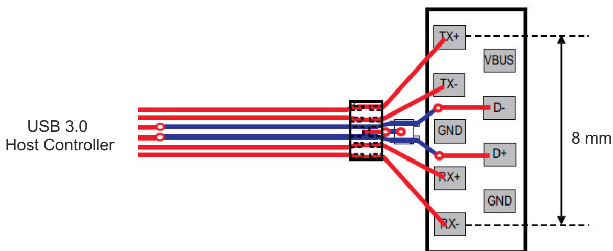
图 9-9. 直通布线
