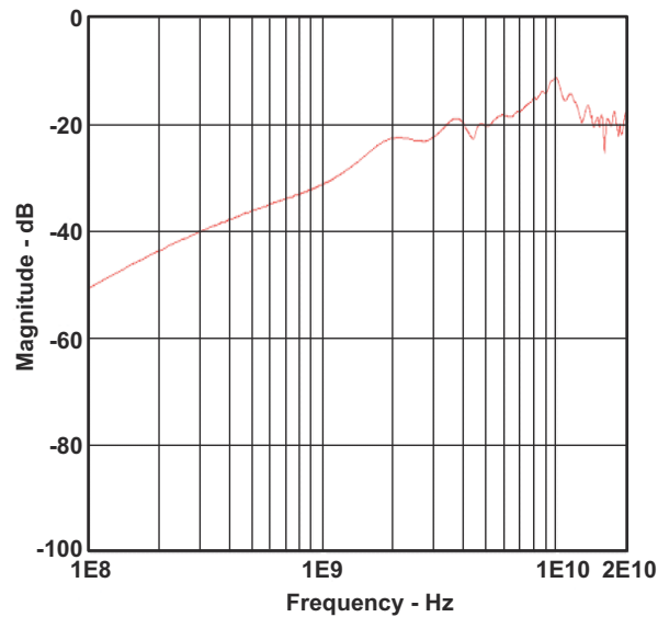
图 9-7. OF Isolation
