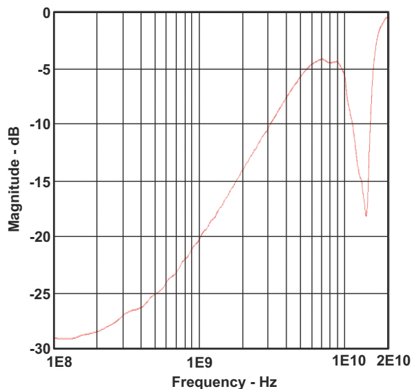
图 6-2. Return Loss
