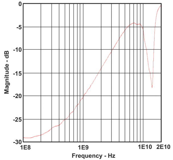
图 9-6. Return Loss
