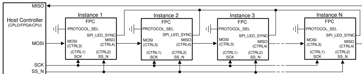
图 7-6. FPC202 Connection Diagram For SPI Mode
