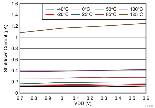
图 5-7. Shutdown Mode I_{DD} vs V_{DD}
