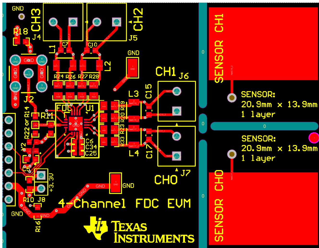
图 7-9. Example PCB Layout: Top Layer (Signal)
