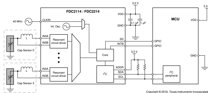
简化原理图
