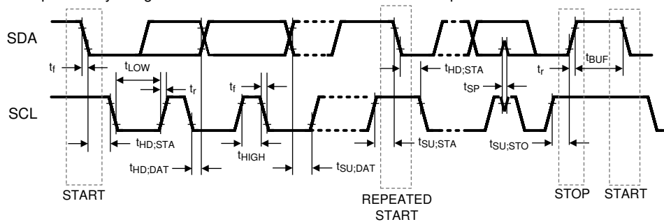
图 5-1. I 2 C Timing
