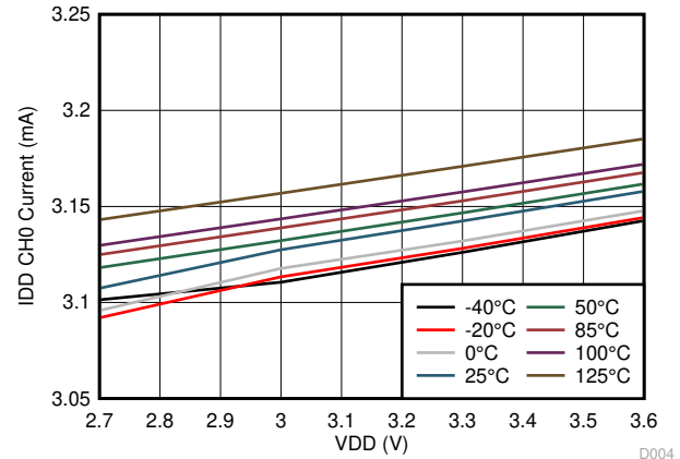
图 5-3. Active Mode I_{DD} vs V_{DD}
