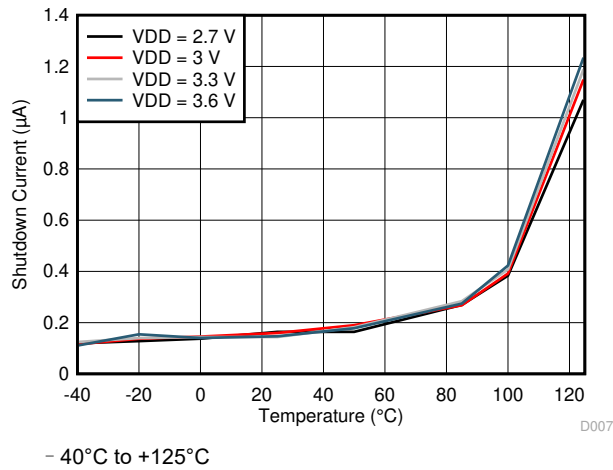
图 5-6. Shutdown Mode I_{DD} vs Temperature
