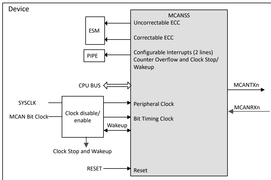
图 6-66. MCAN 模块概述
