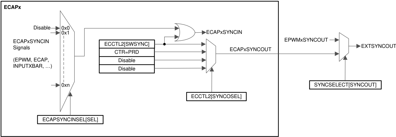
图 6-55. eCAP 同步方案
