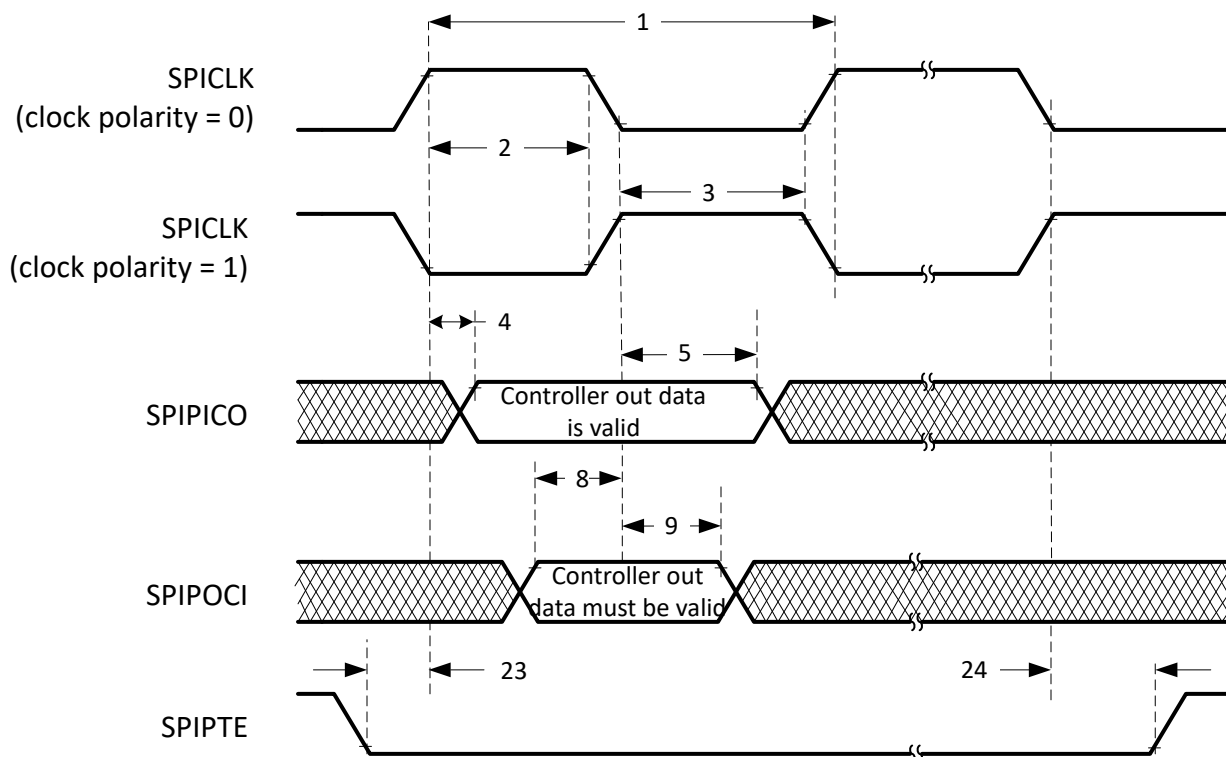
图 6-78. SPI 控制器模式外部时序 (时钟相位 = 0)
