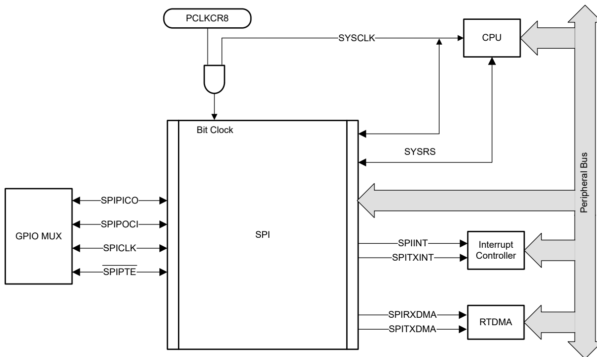
图 6-77. SPI CPU 接口
