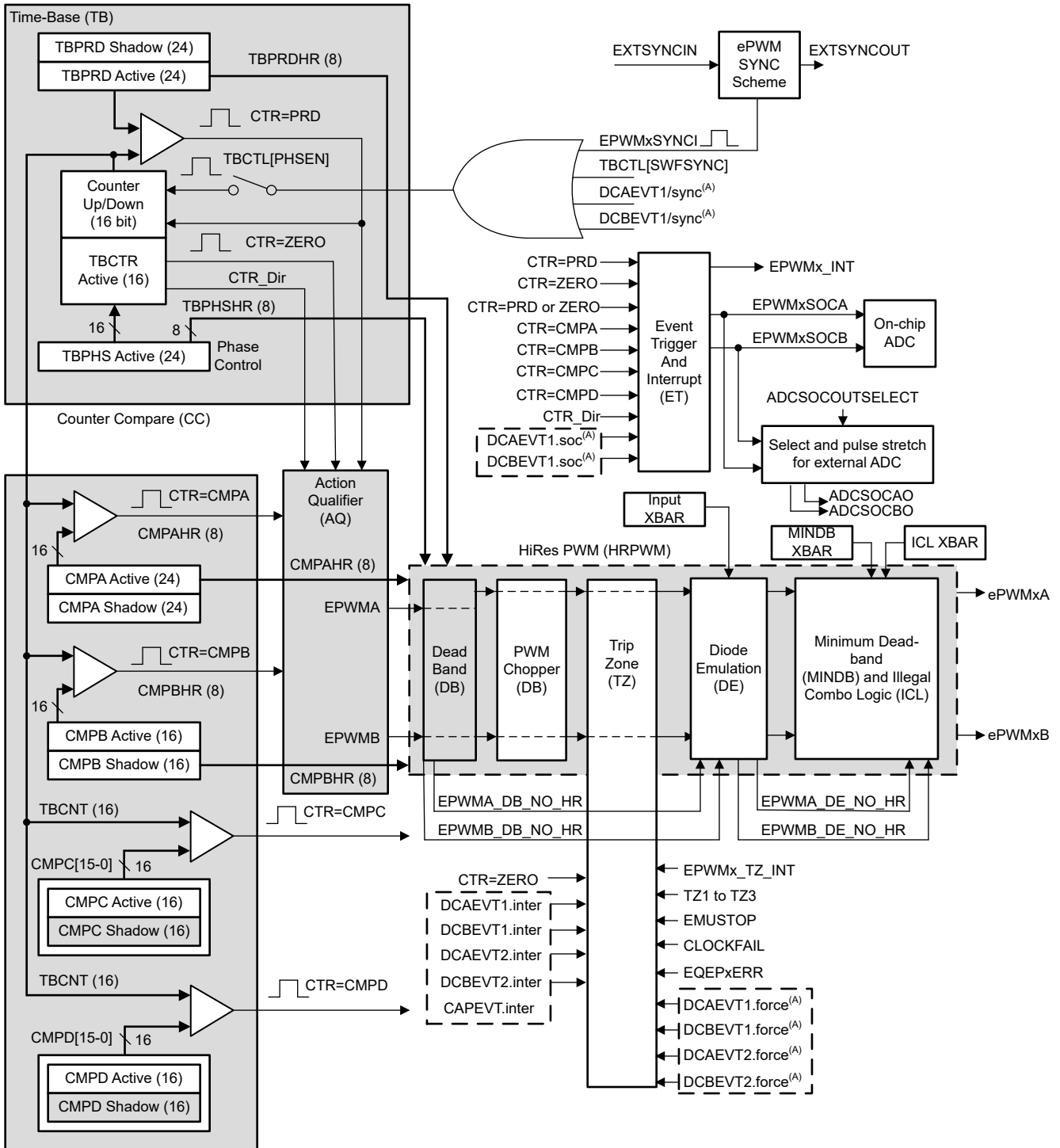
图 6-58. ePWM 子模块和关键内部信号互连
