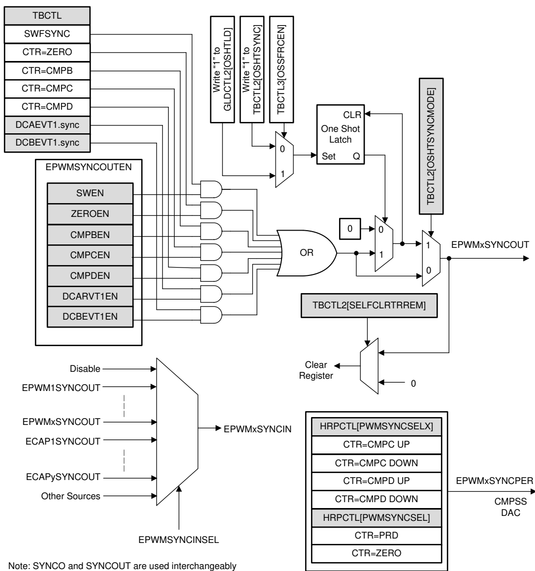
图 6-60. 同步链架构
