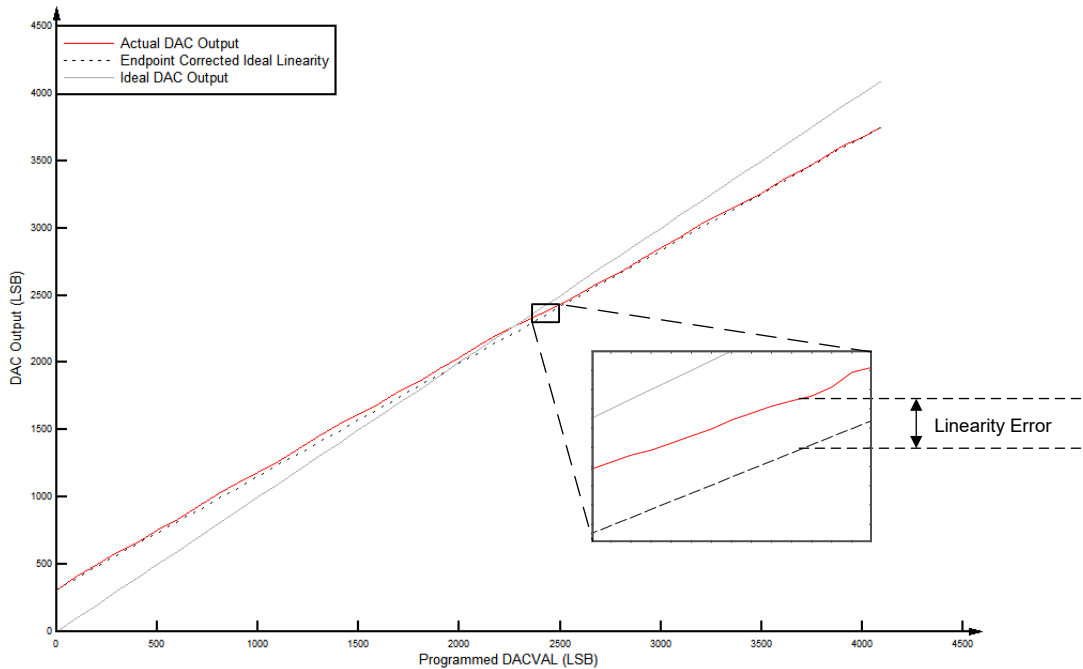
图 6-52. CMPSS DAC 静态线性
