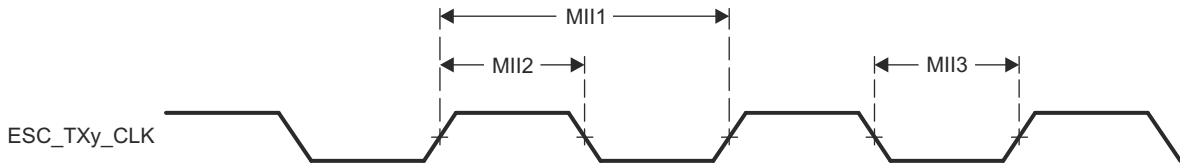
图 6-84. EtherCAT 发送时钟时序 ( MII 运行模式 )
