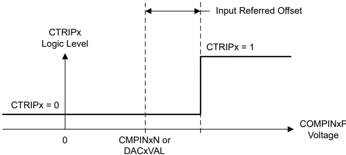
图 6-48. CMPSS 比较器以输入为基准的偏移量
