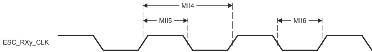
图 6-86. EtherCAT 接收时钟时序 ( MII 运行模式 )
