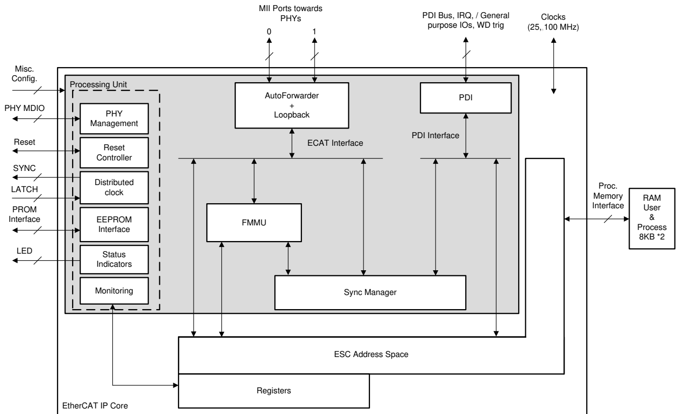
图 6-83. EtherCAT IP 方框图
