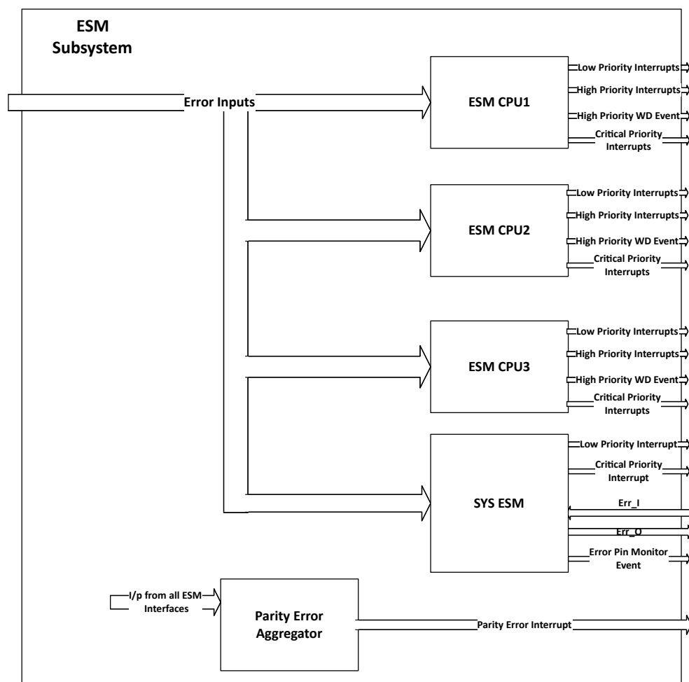
图 7-2. ESM-SS 方框图
