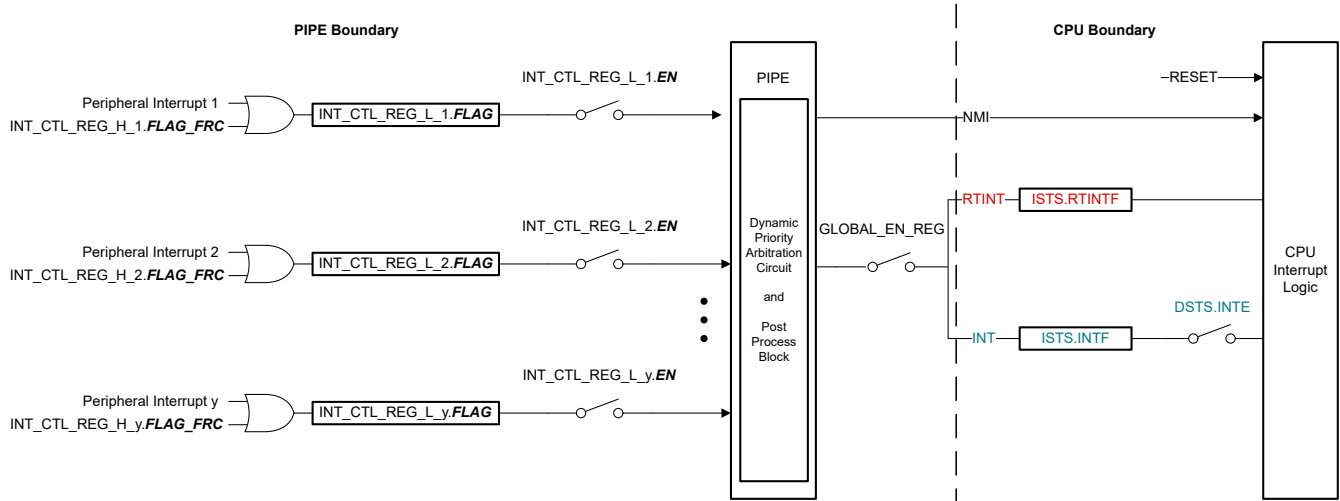
图 7-15. 中断传播
