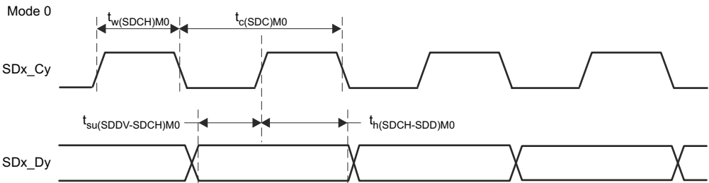
图 6-65. SDFM 时序图 - 模式 0
