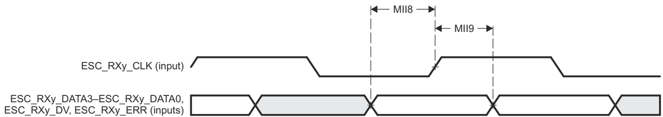
图 6-87. EtherCAT 接收接口时序 ( MII 运行模式 )
