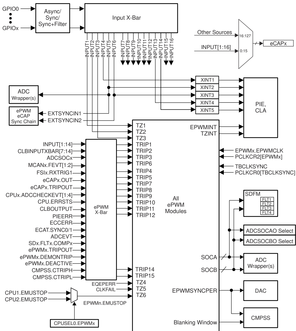
图 6-59. ePWM 跳变输入连接
