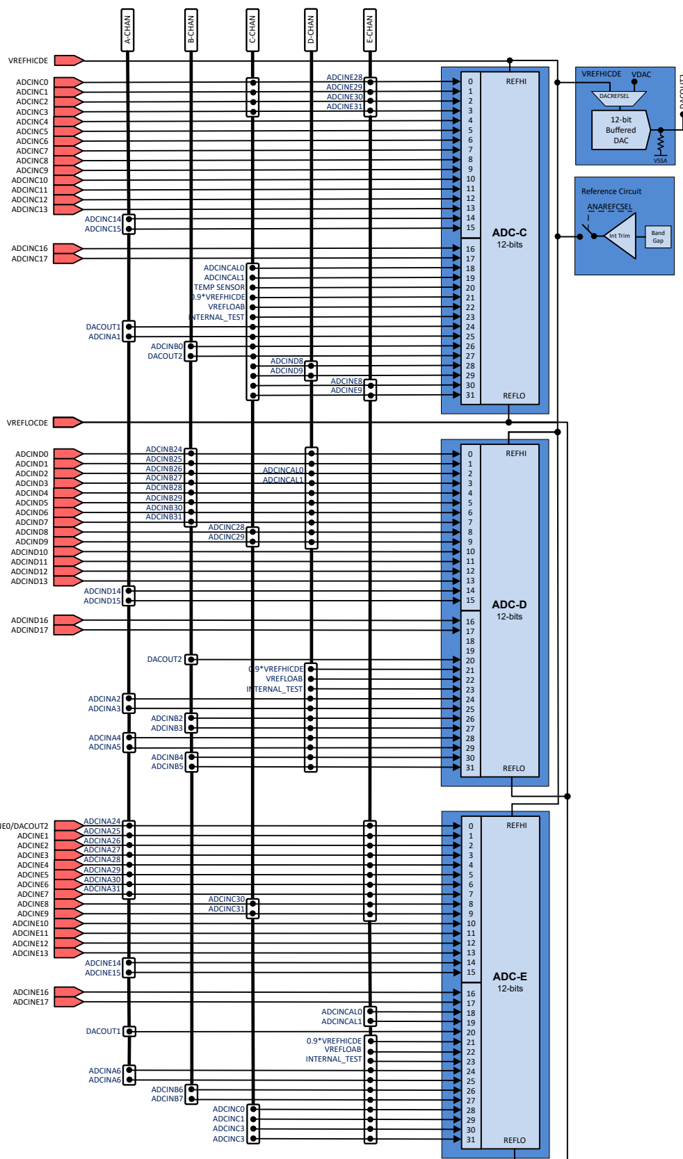
图 6-33. 模拟子系统方框图 ( ADC C、ADC D 和 ADC E )
