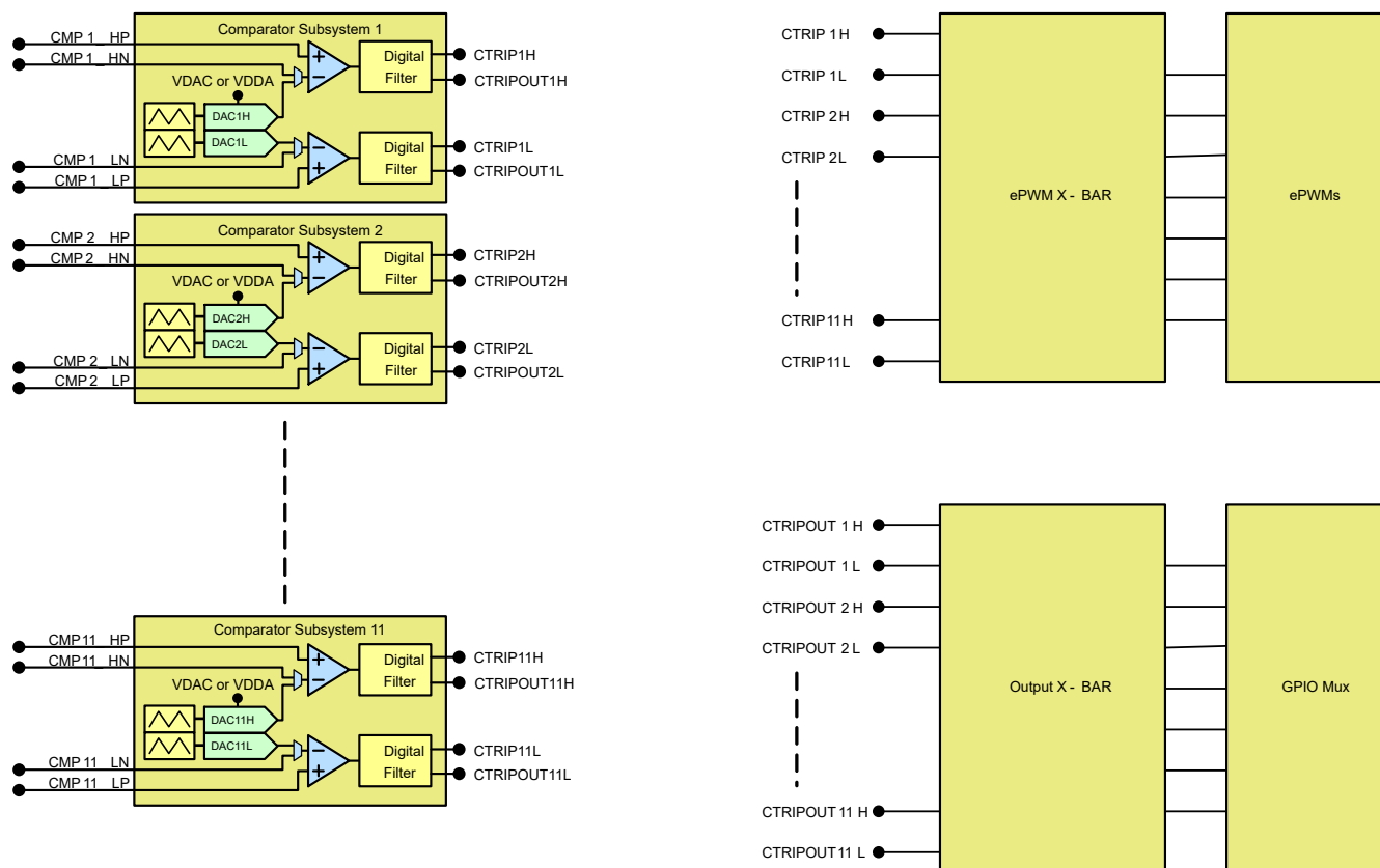
图 6-45. CMPSS 连接
