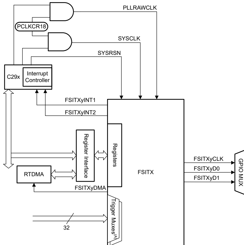
图 6-70. FSIRX CPU 接口
