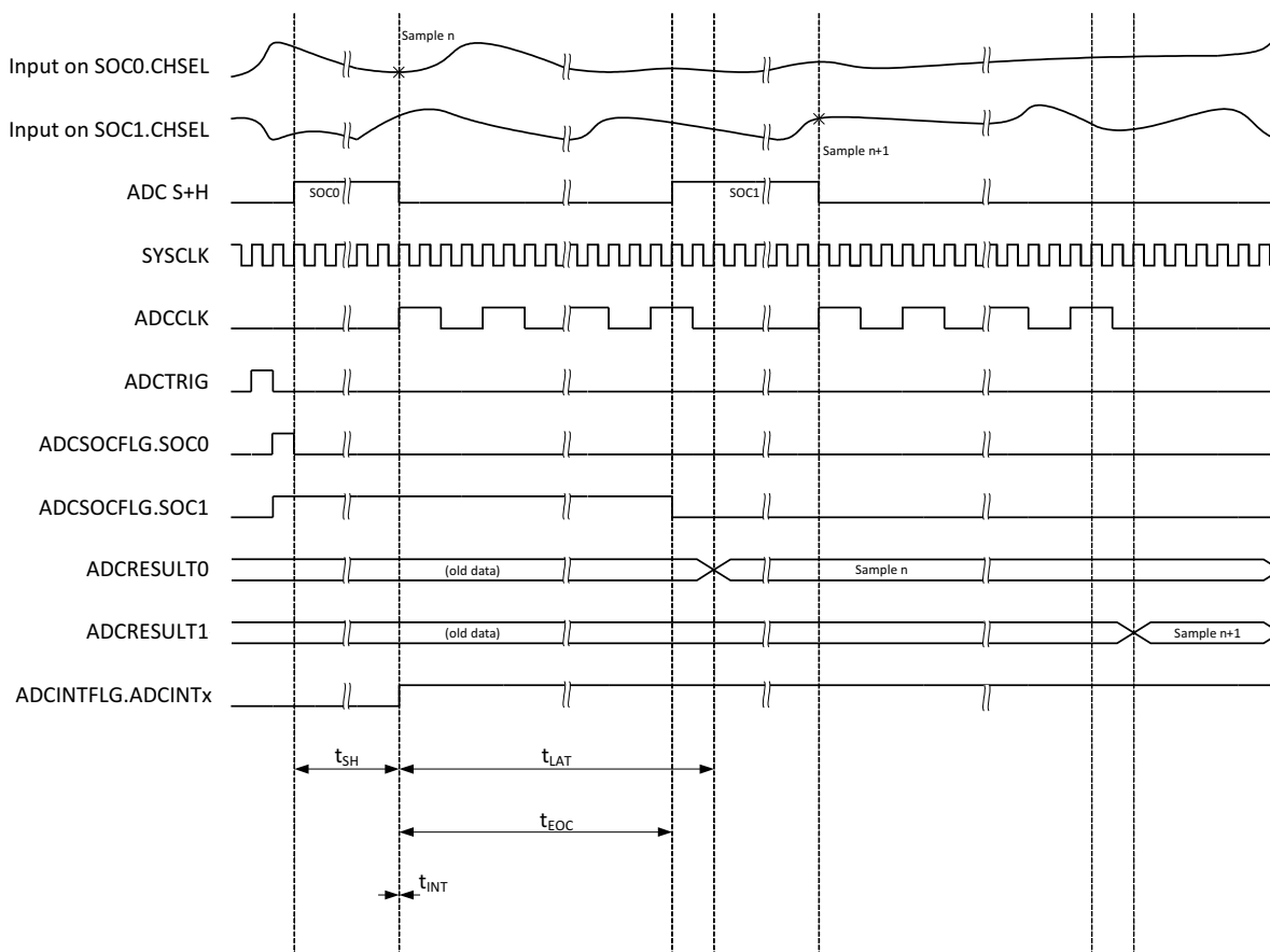
图 6-41. 提前中断模式下 12 位模式的 ADC 时序
