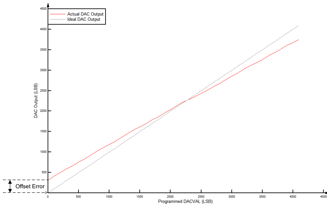
图 6-50. CMPSS DAC 静态偏移量
