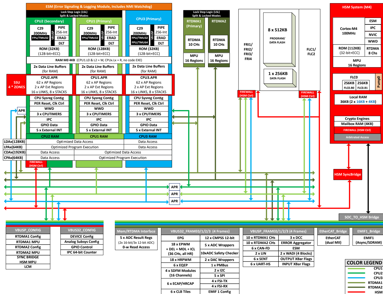
图 3-1. 功能方框图
