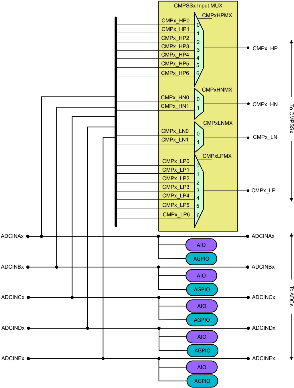
图 6-34. 模拟组连接
