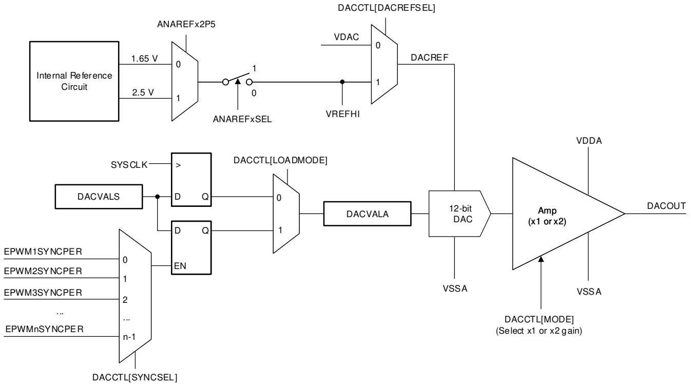
图 6-53. DAC 模块方框图
