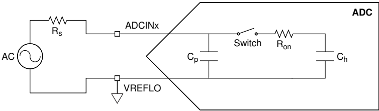
图 6-39. 单端输入模型
