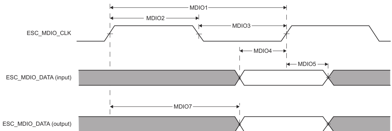
图 6-88. EtherCAT MDIO 时序图
