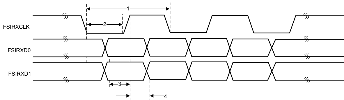
图 6-72. FSIRX 时序
