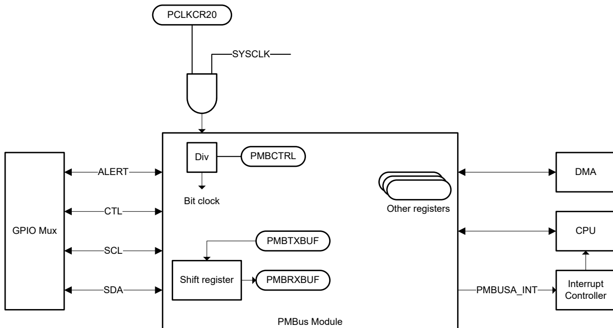
图 6-76. PMBus 方框图
