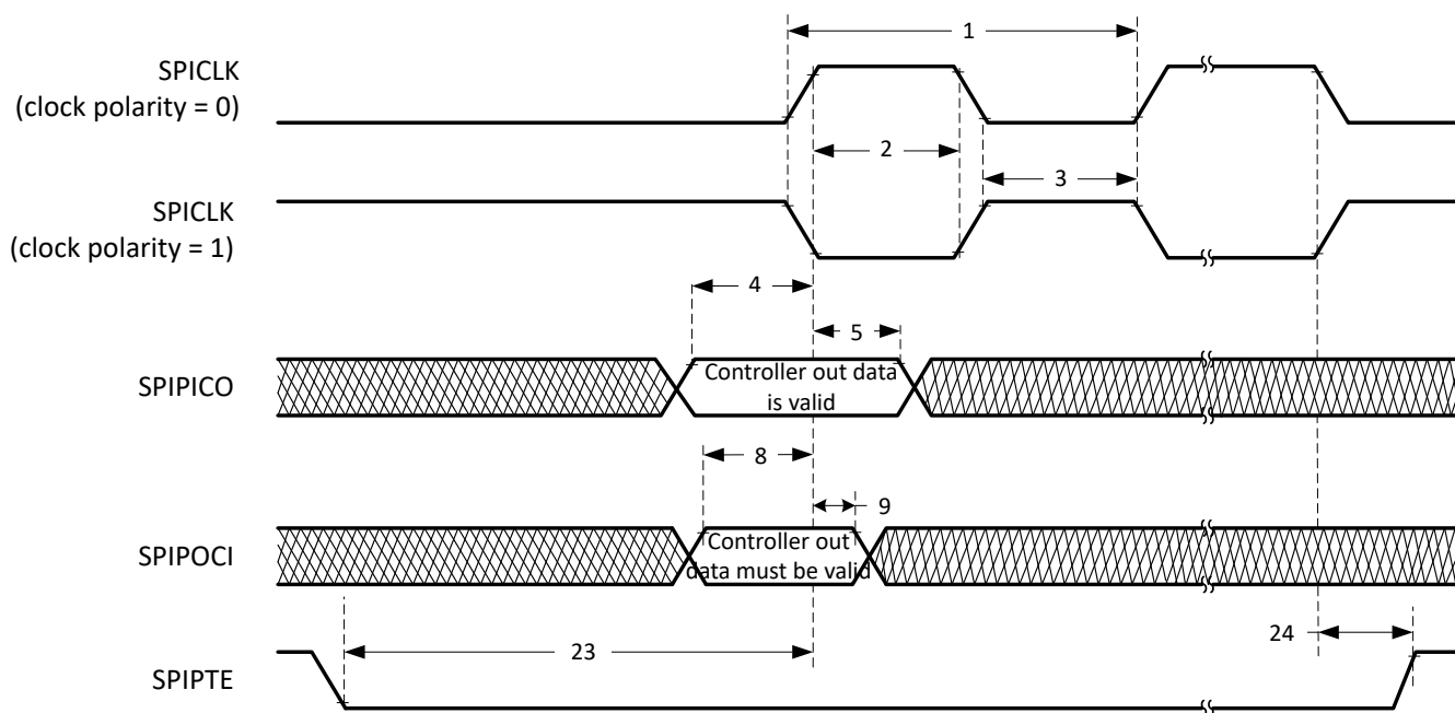
图 6-78. SPI 控制器模式外部时序 (时钟相位 = 0)
