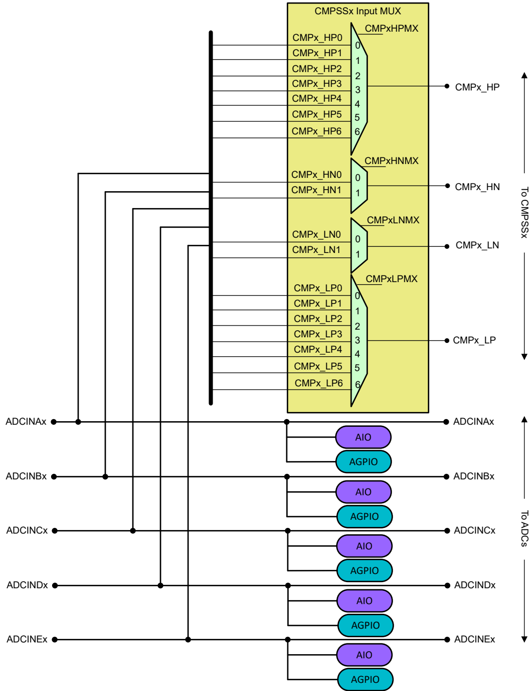
图 6-34. 模拟组连接
