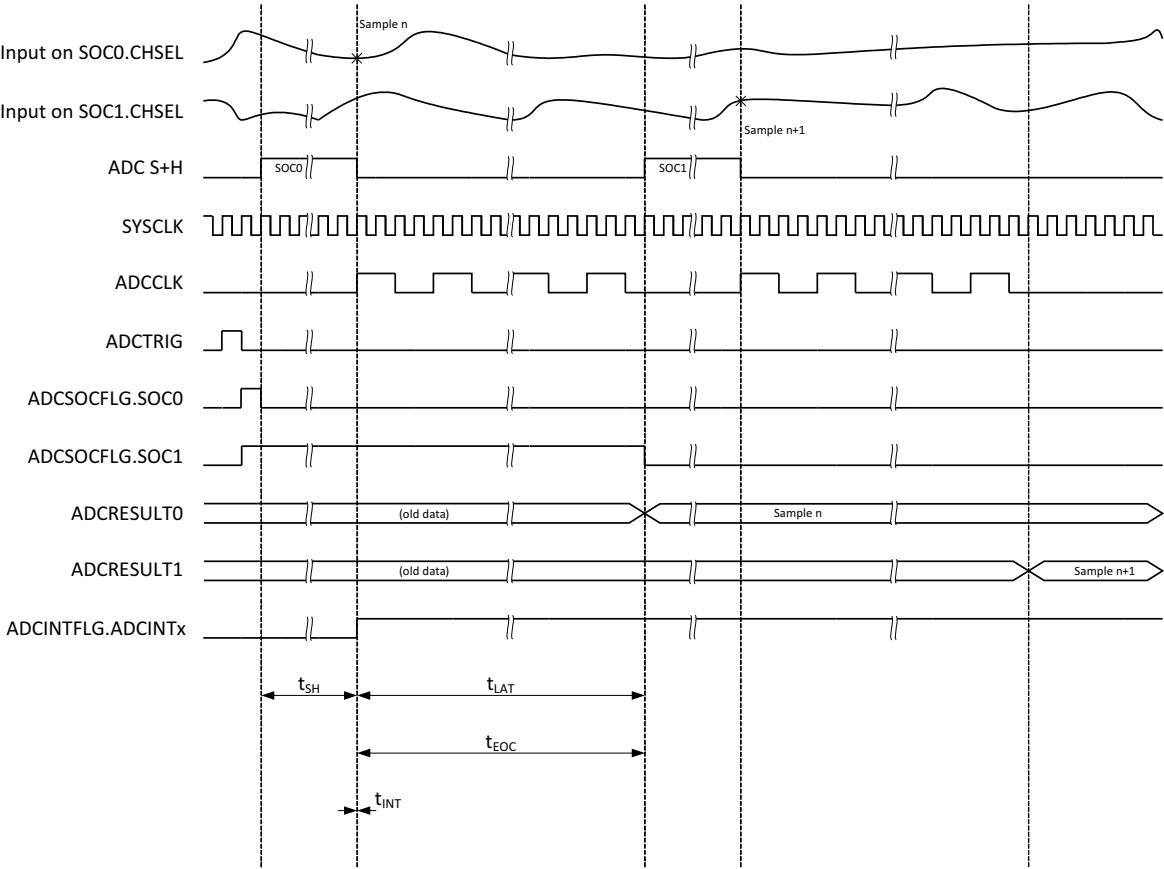
图 6-43. 提前中断模式下 16 位模式的 ADC 时序
