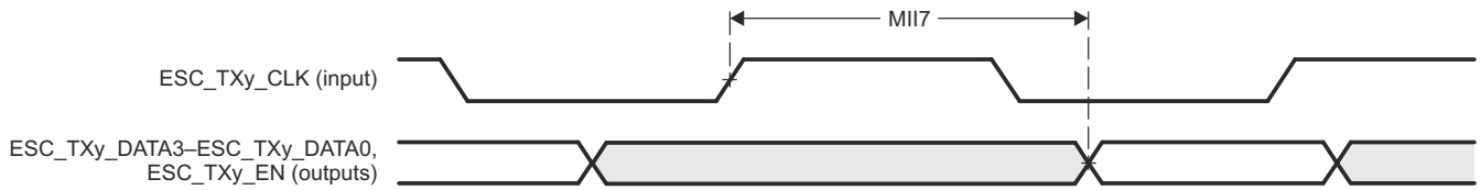
图 6-85. EtherCAT 发送接口时序 ( MII 运行模式 )
