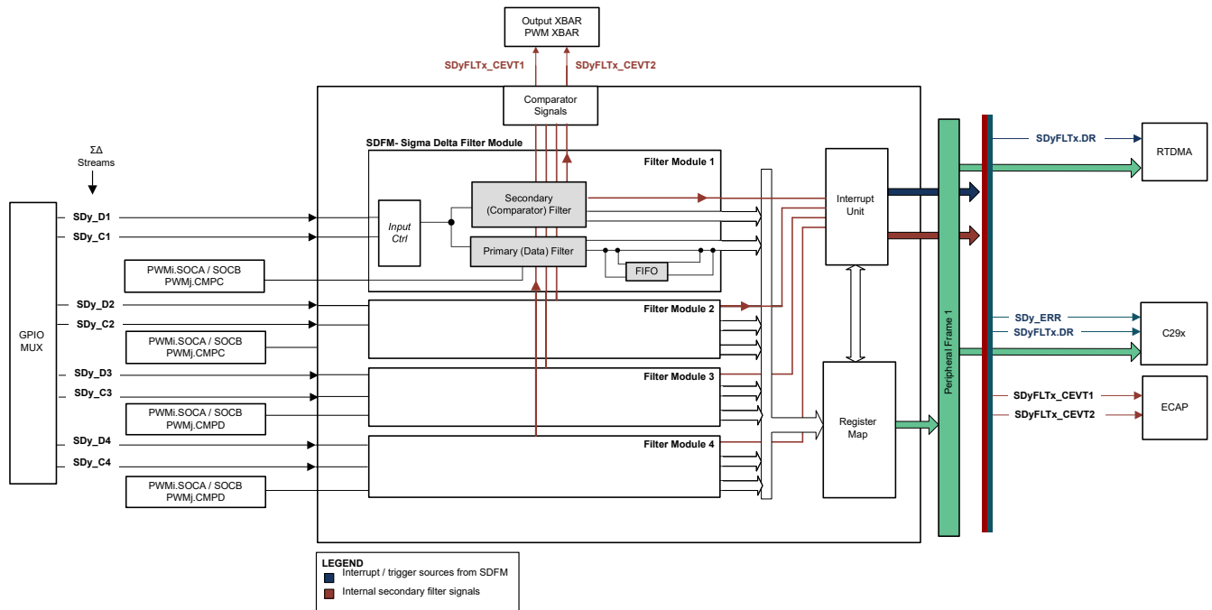
图 6-64. \Sigma - \Delta 滤波器模块 (SDFM) 方框图
