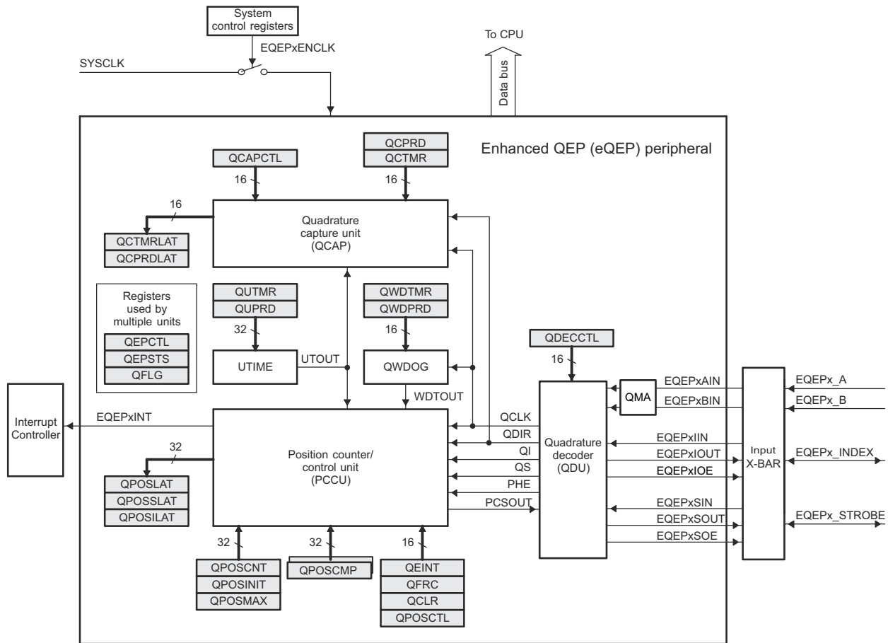
图 6-63. eQEP 方框图
