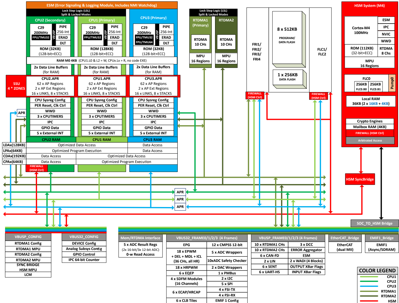
图 7-1. 功能方框图
