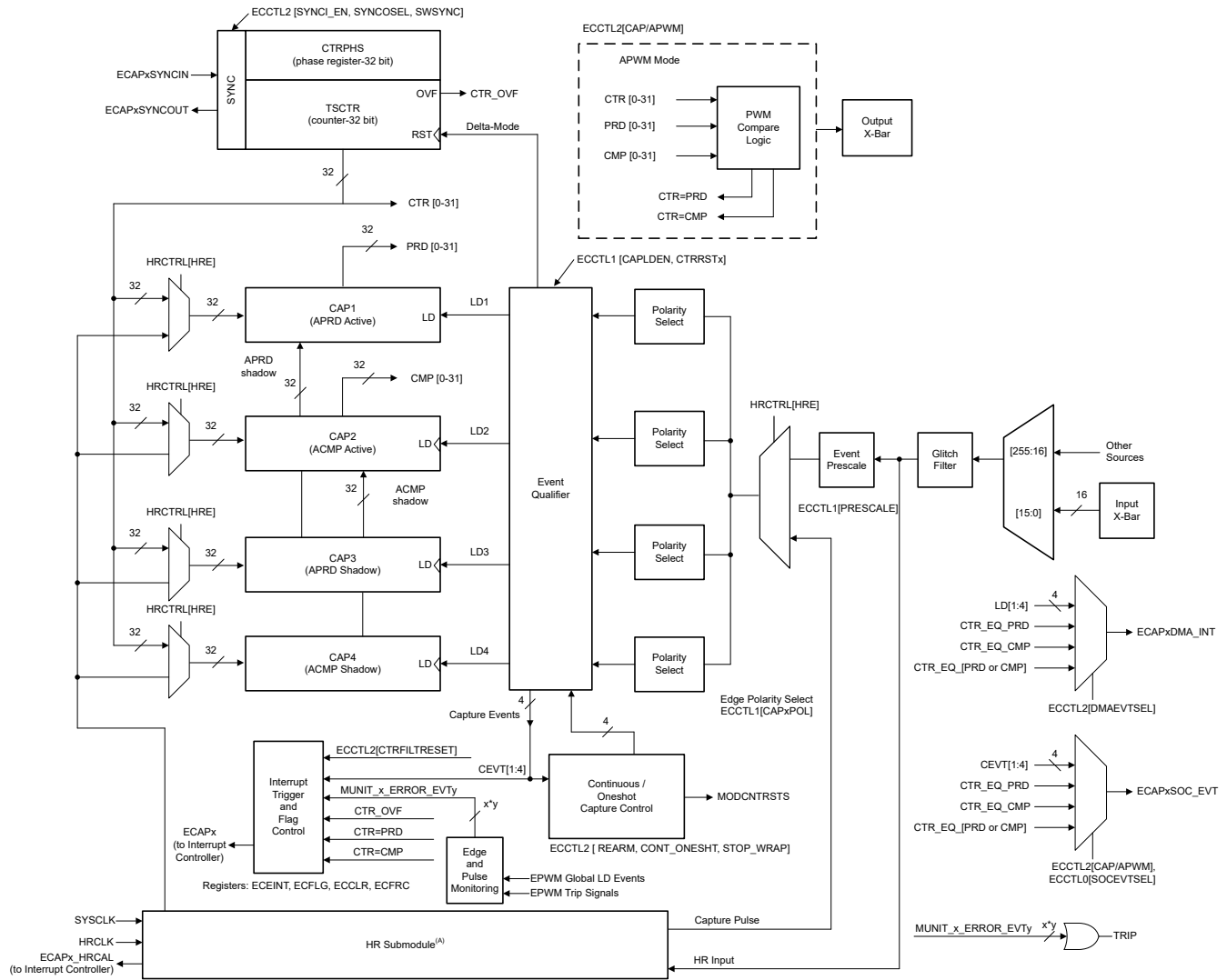
图 6-54. eCAP 方框图
