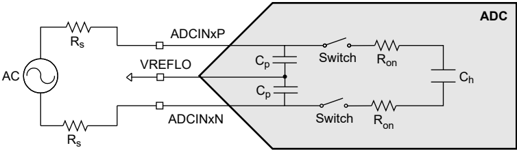
图 6-40. 差分输入模型
