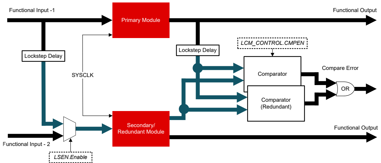
图 7-22. LCM 方框图
