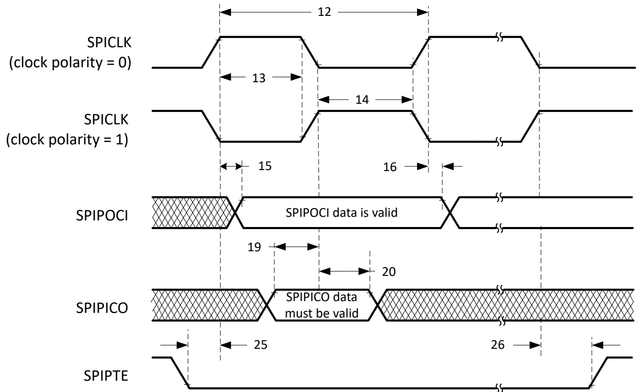
图 6-80. SPI 外设模式外部时序 ( 时钟相位 = 0 )
