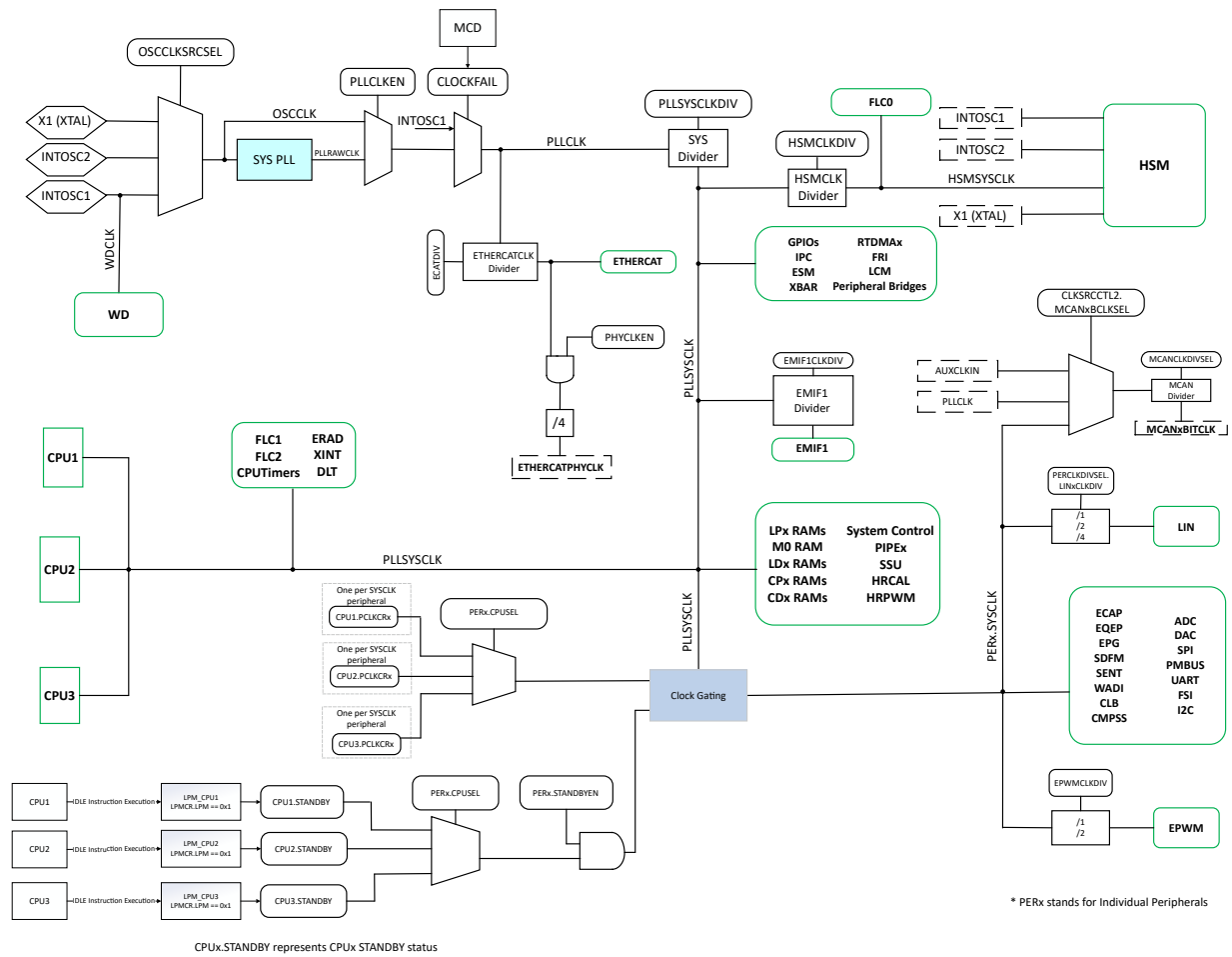
图 6-9. 计时系统
