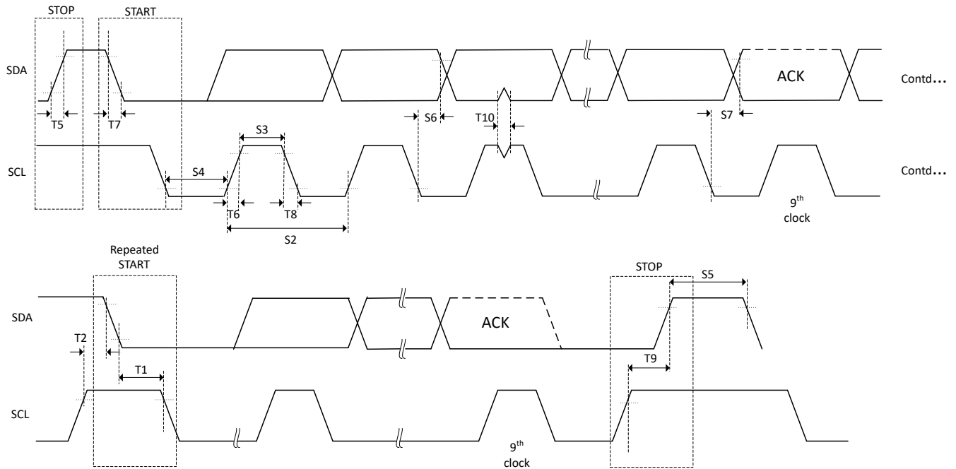
图 6-75. I2C 时序图
