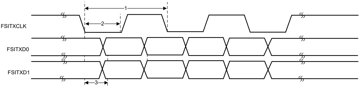
图 6-69. FSITX 时序
