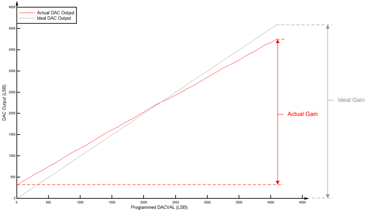
图 6-51. CMPSS DAC 静态增益
