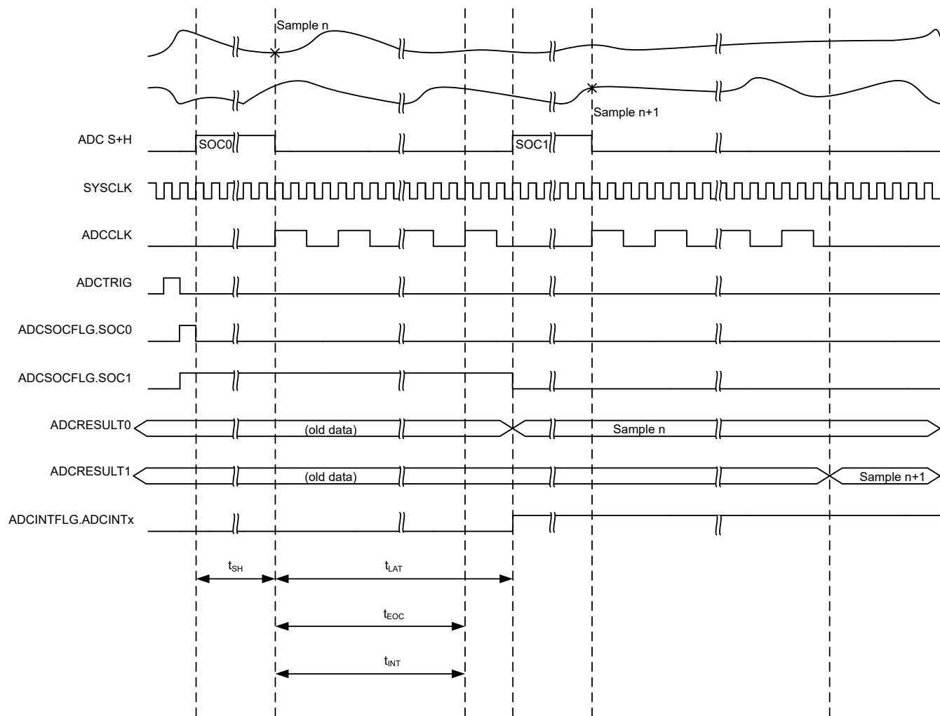
图 6-44. 后期中断模式下 16 位模式的 ADC 时序 ( SYSCLK 周期 )
