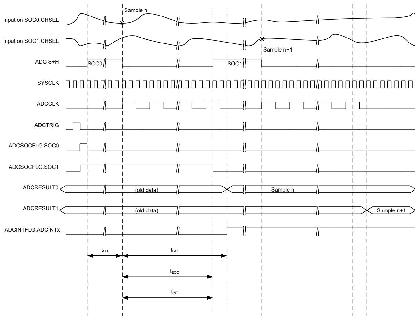
图 6-42. 后期中断模式下 12 位模式的 ADC 时序
