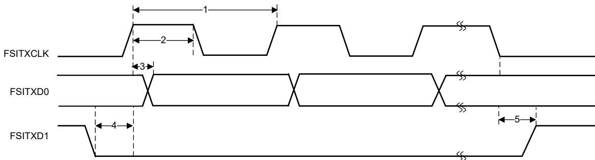
图 6-73. FSITX SPI 信令模式时序
