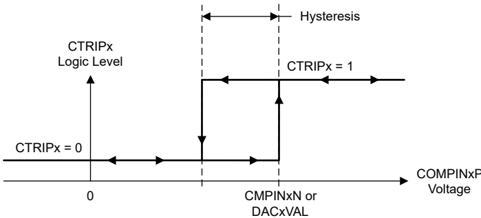
图 6-49. CMPSS 比较器迟滞
