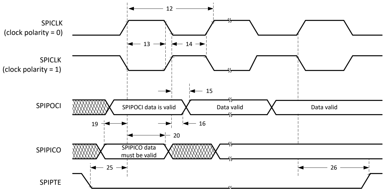
图 6-81. SPI 外设模式外部时序 ( 时钟相位 = 1 )
