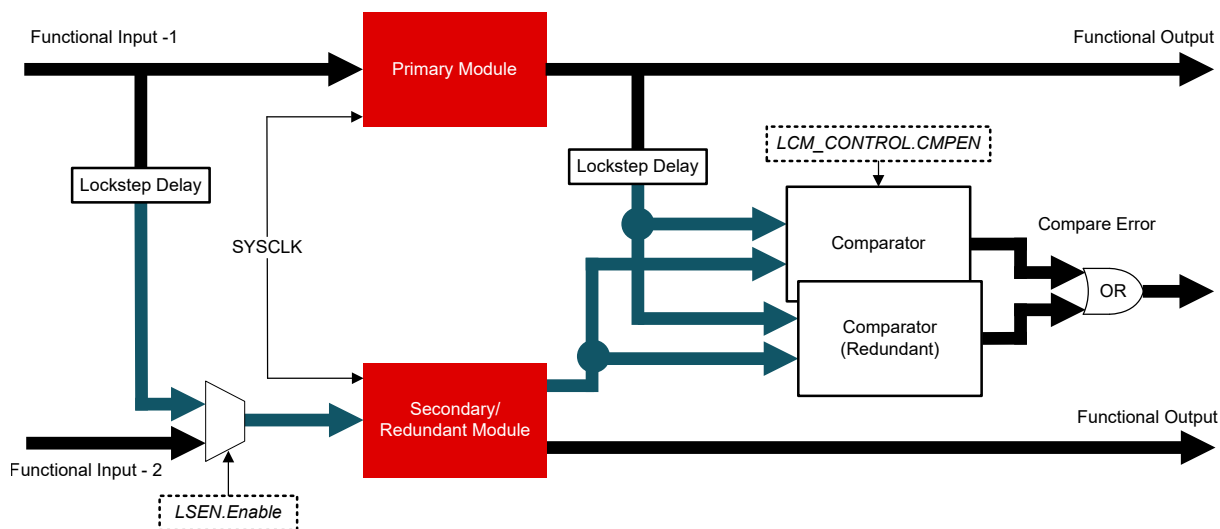
图 7-22. LCM 方框图
