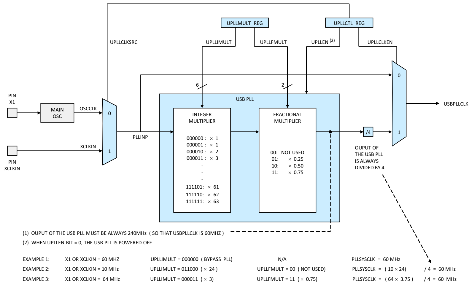
图 6-9. USB PLL
