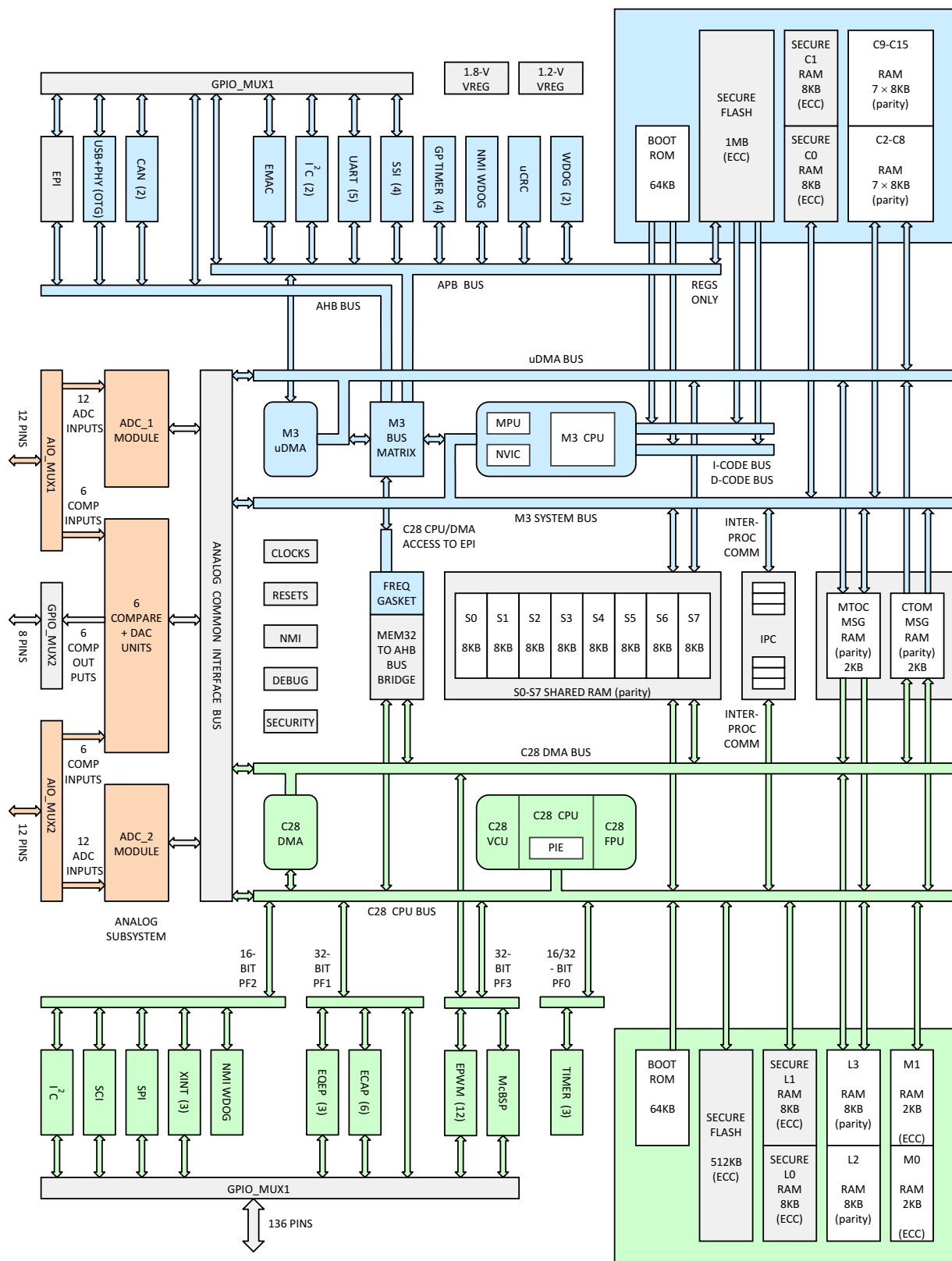
图 1-1. 功能框图
