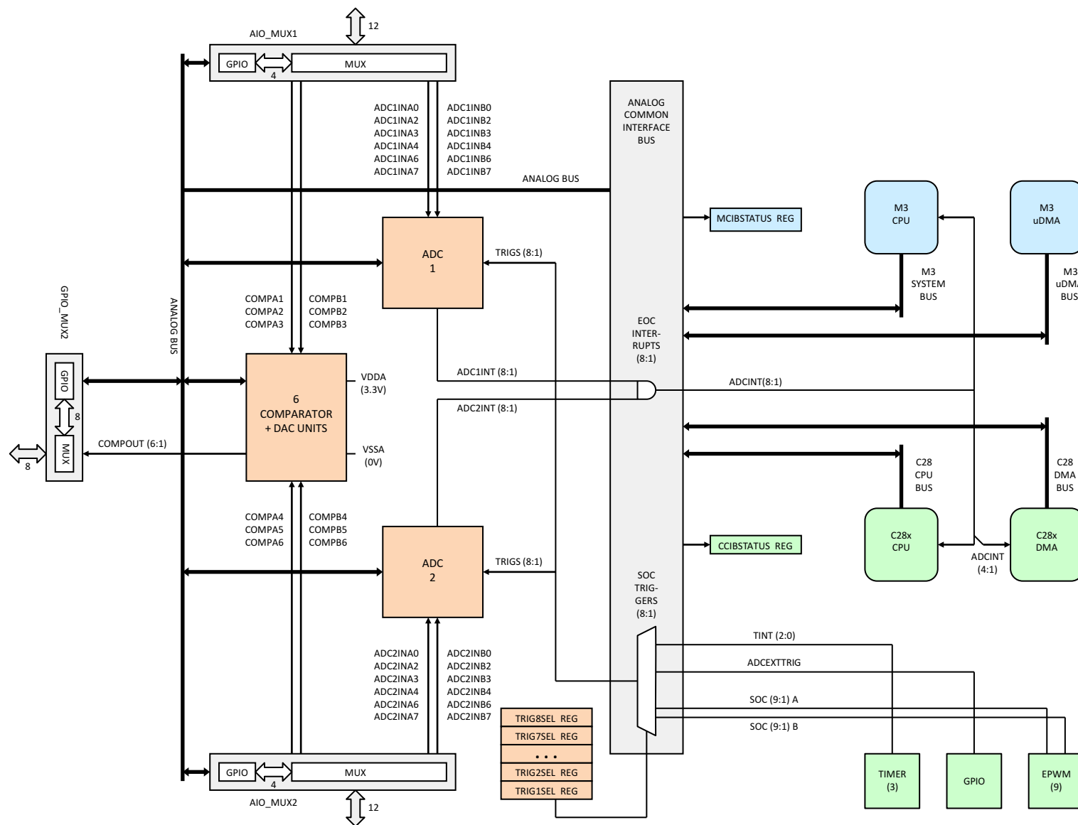
图 6-3. Analog Subsystem
