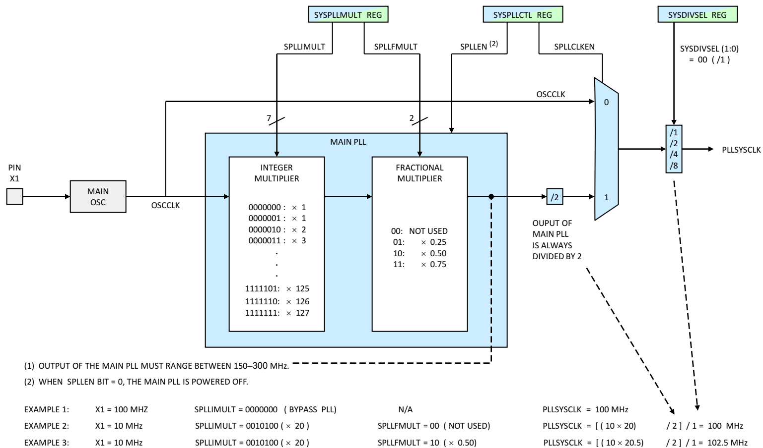
图 6-8. Main PLL
