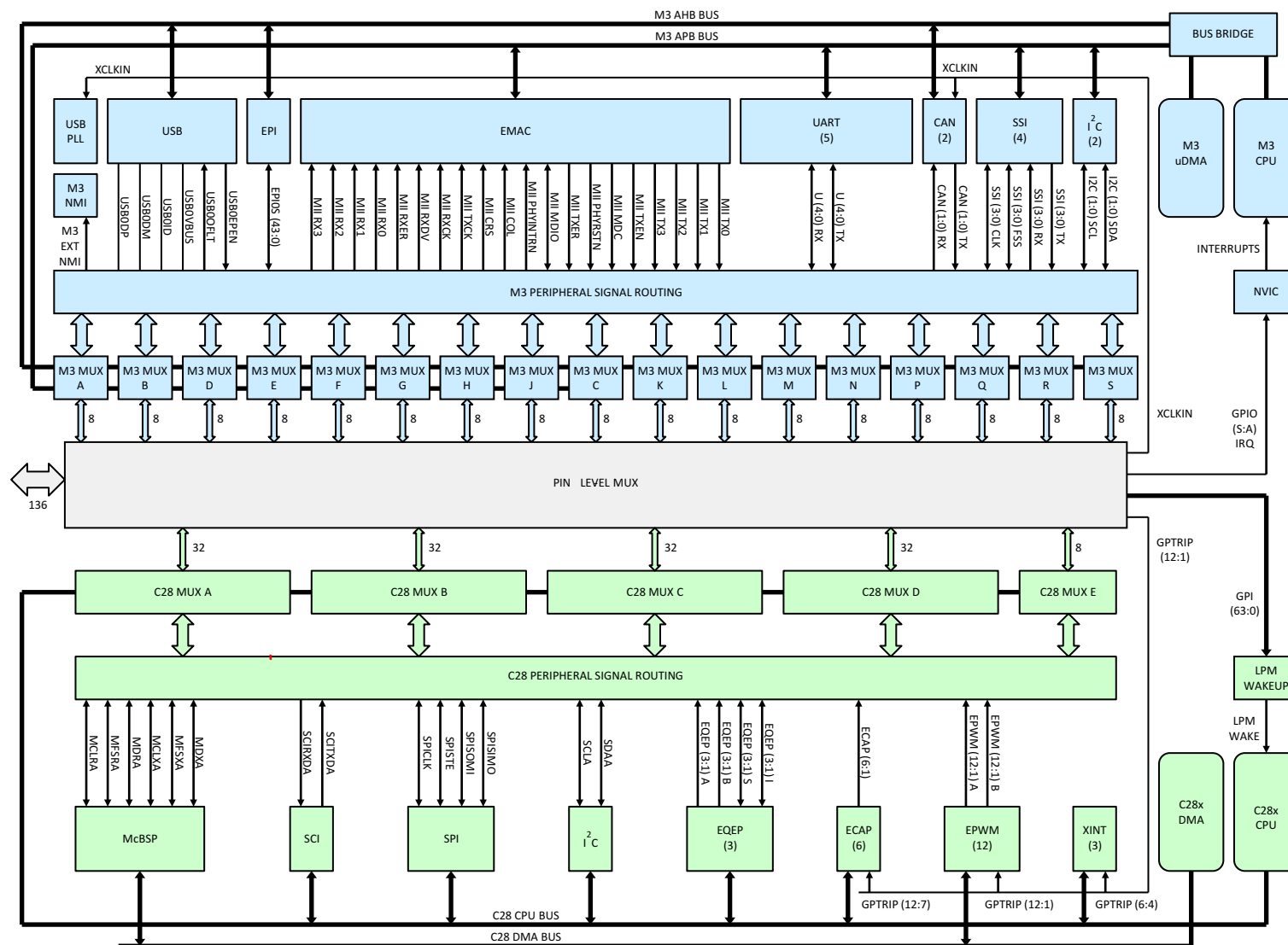
图 6-15. GPIO_MUX1 Block
