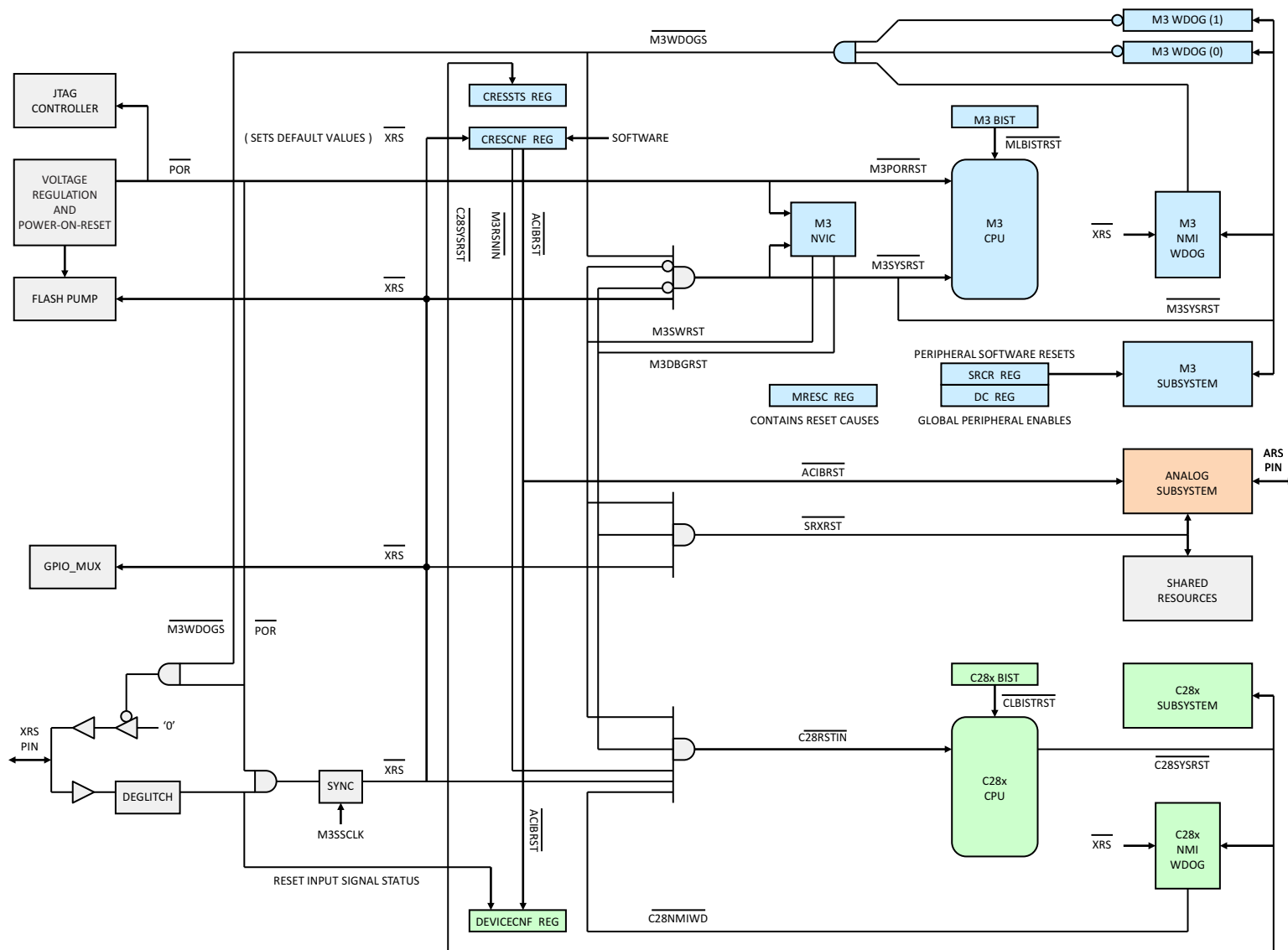
图 6-5. Resets
