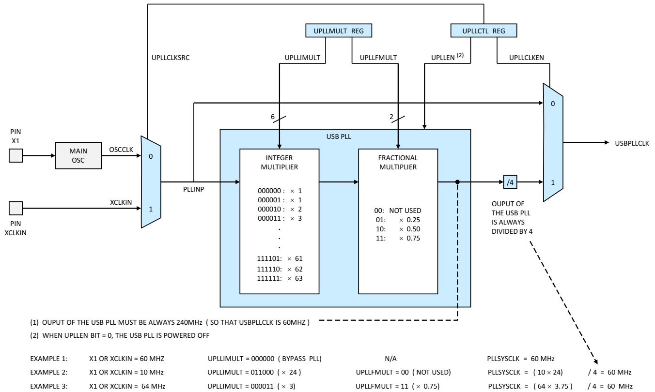
图 8-9. USB PLL
