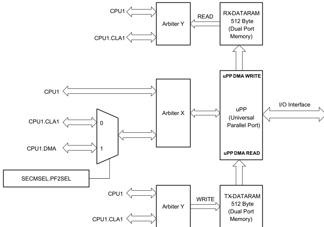
图 6-80. uPP 集成
