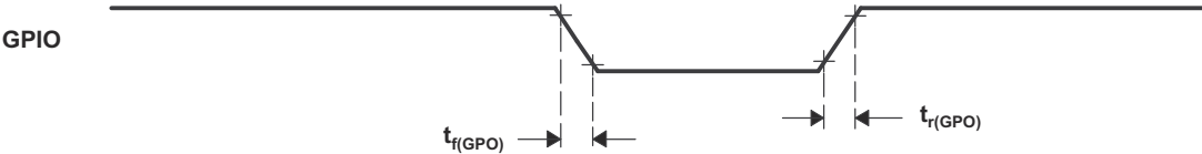
图 6-17. 通用输出时序
