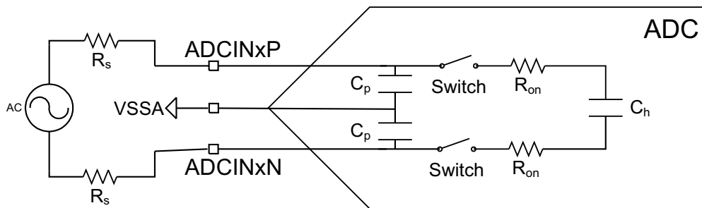
图 6-36. 差分输入模型
