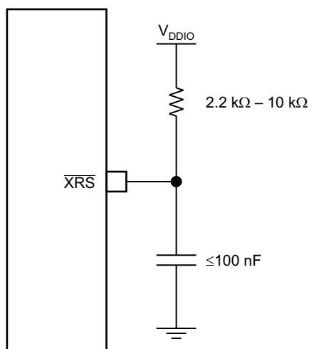
图 6-5. 复位电路
