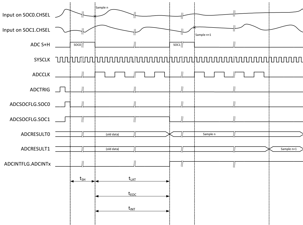
图 6-39. 16 位模式的 ADC 时序
