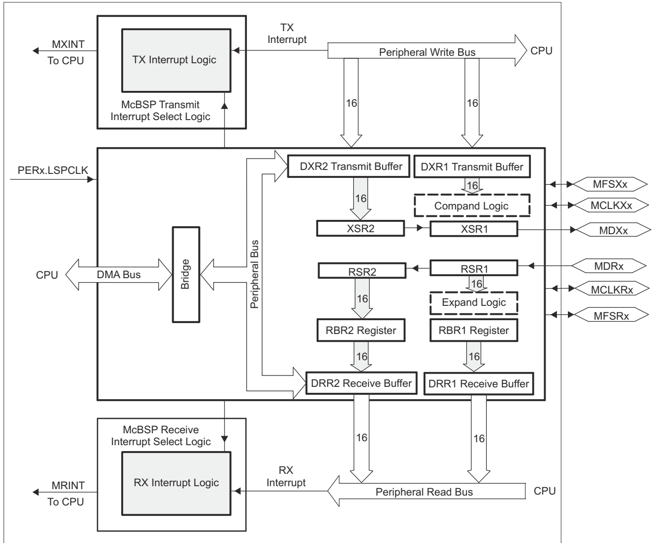
图 6-66. McBSP 方框图
