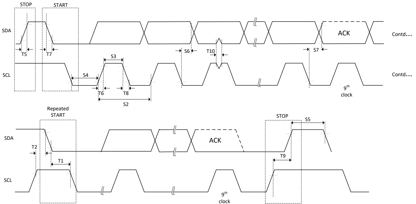
图 6-65. I2C 时序图
