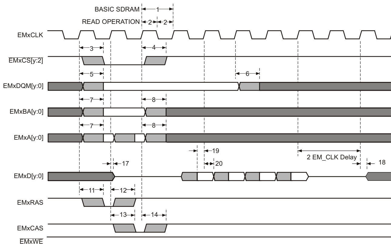
图 6-30. 基本 SDRAM 读取操作
