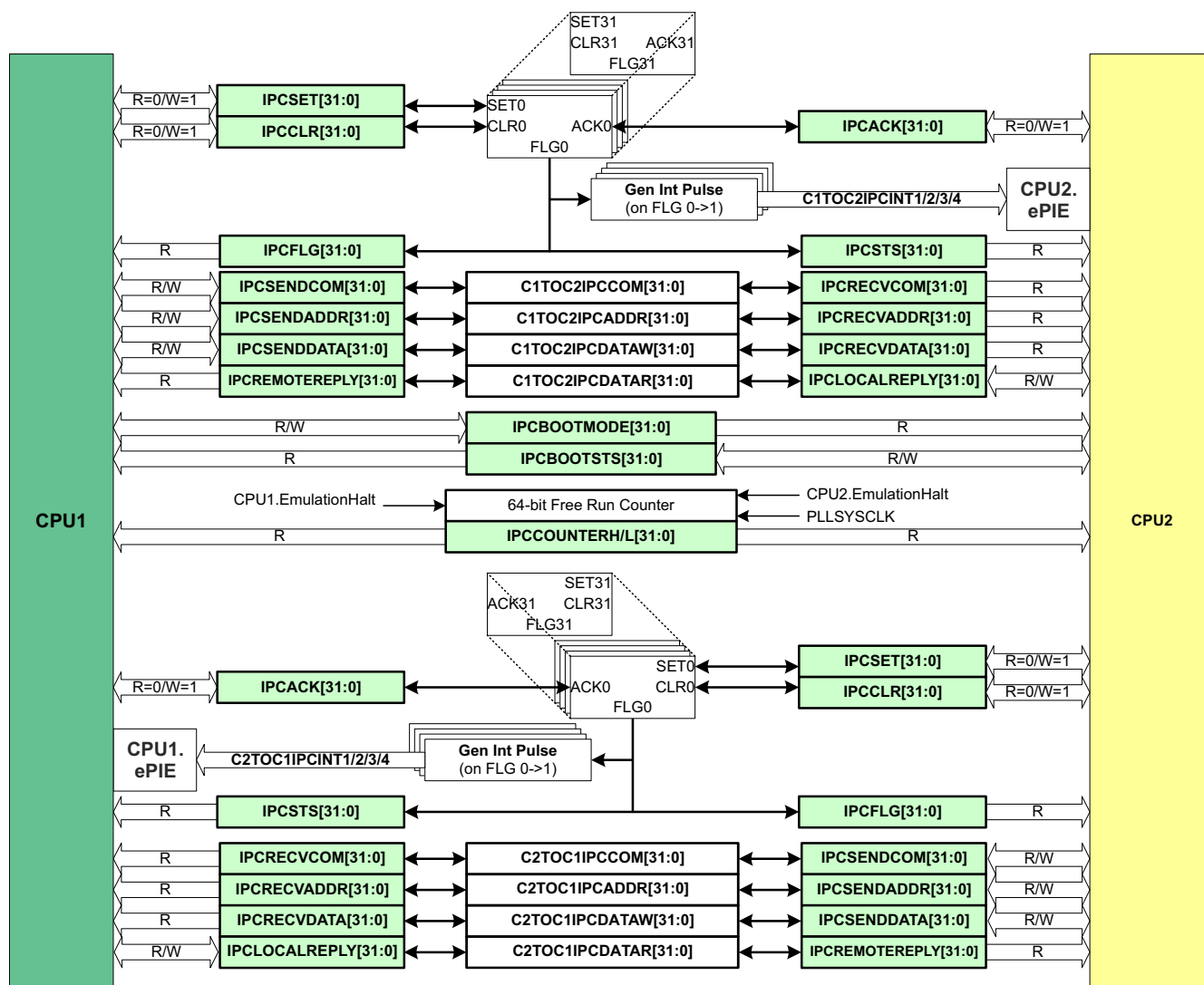
图 7-4. IPC 架构
