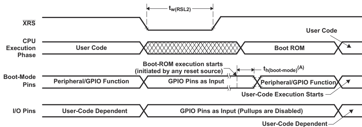
图 6-6. 上电复位
