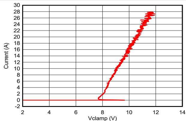
图 5-6. 正 TLP 曲线
