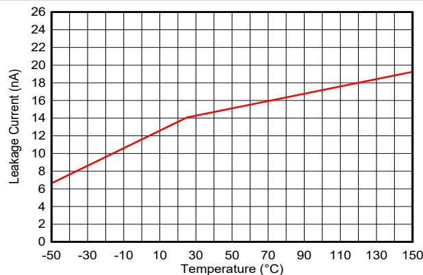
图 5-5. 漏电流与温度间的关系
