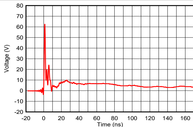
图 5-1. +8kV IEC 61000-4-2 钳位电压波形
