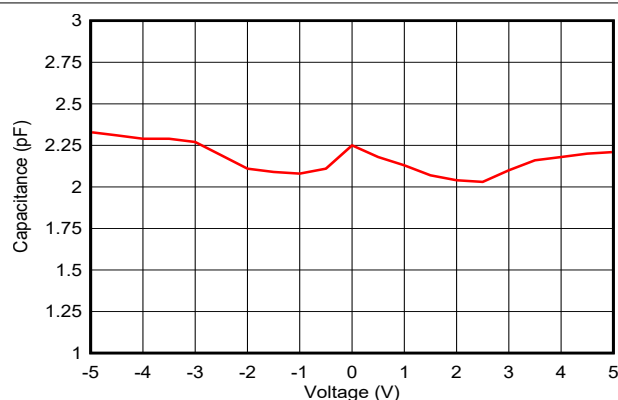
图 5-3. 电容与偏置电压间的关系
