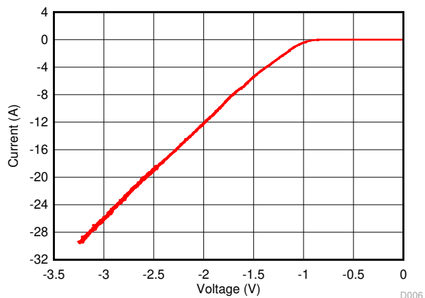
图 5-4. DC I-V Curve
