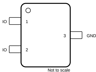
图 4-1. DBZ 或 DCK 封装， SOT-23 ( 顶视图 )
