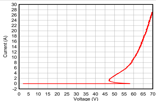
图 5-7. 正 TLP 曲线
