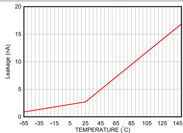
图 5-6. 漏电流与温度之间的关系
