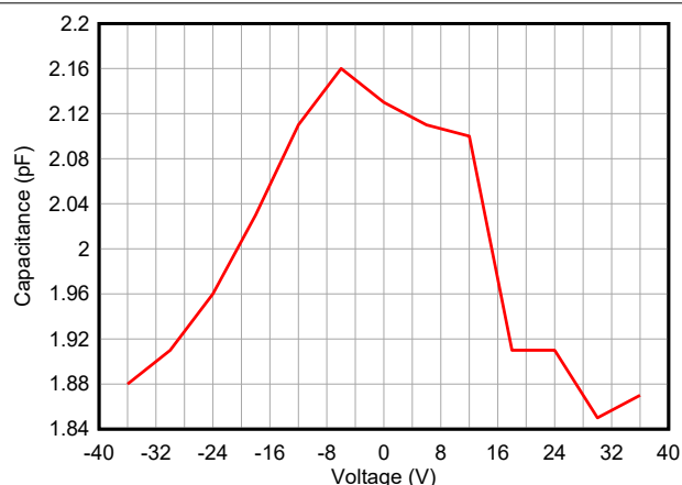
图 5-11. 电容与偏置电压间的关系
