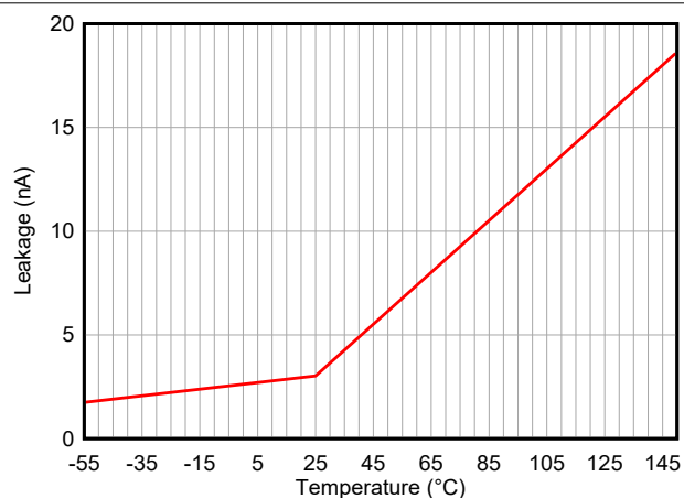
图 5-12. 漏电流与温度之间的关系
