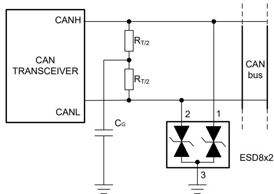
ESD8x2 典型应用
