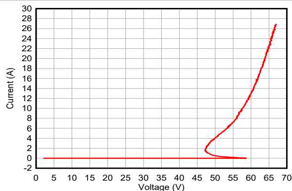
图 5-1. 正 TLP 曲线
