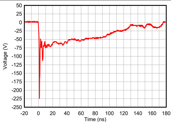
图 5-4. -8kV 钳位 IEC 波形
