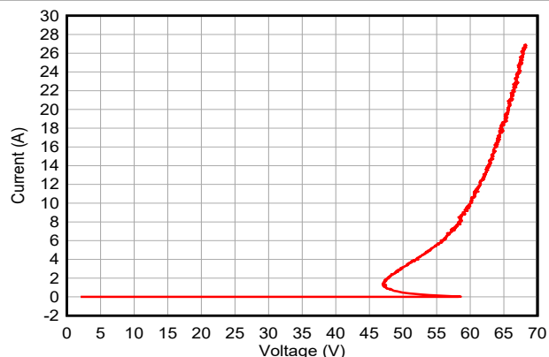
图 5-8. 负 TLP 曲线
