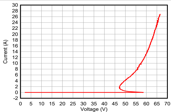
图 5-2. 负 TLP 曲线
