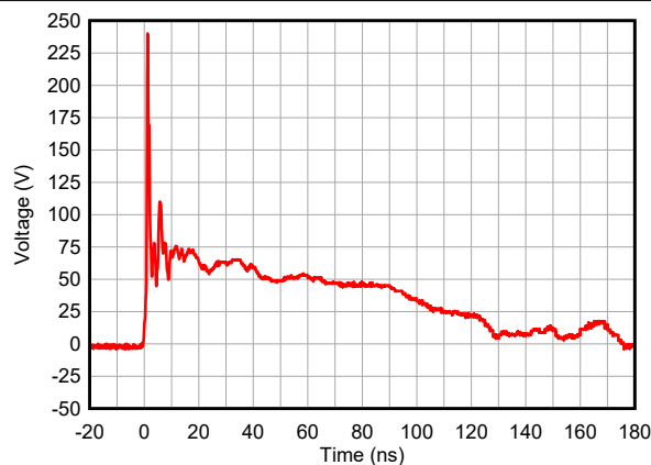
图 5-3. +8kV 钳位 IEC 波形
