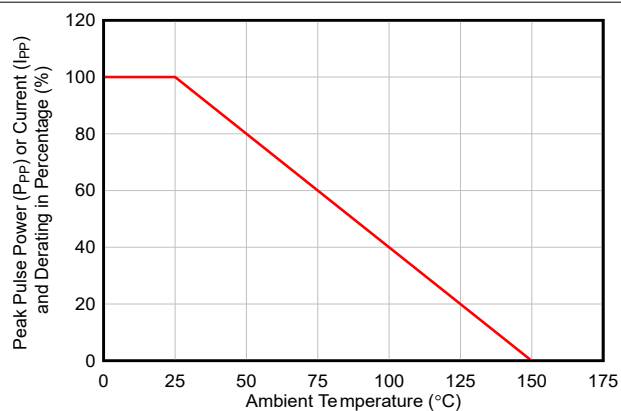
图 5-4. 峰值脉冲功率降额曲线
