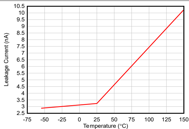
图 5-3. 漏电流与温度间的关系
