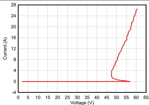
图 5-1. 正 TLP 曲线
