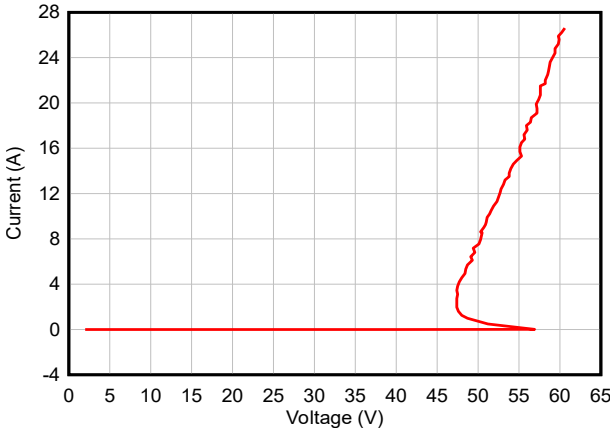
图 5-1. 正 TLP 曲线
