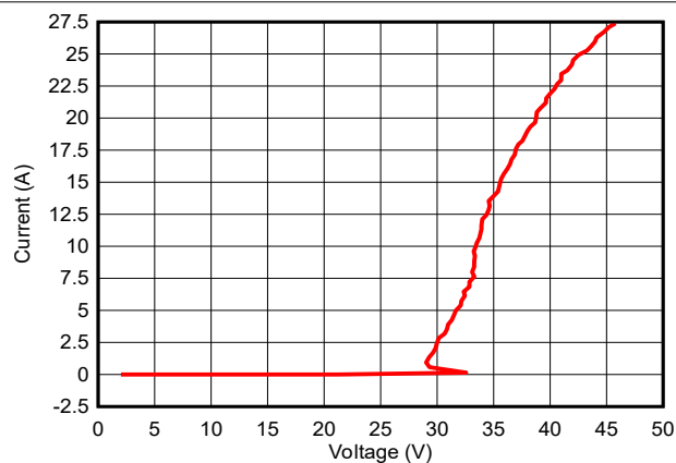
图 5-1. 正 TLP 曲线
