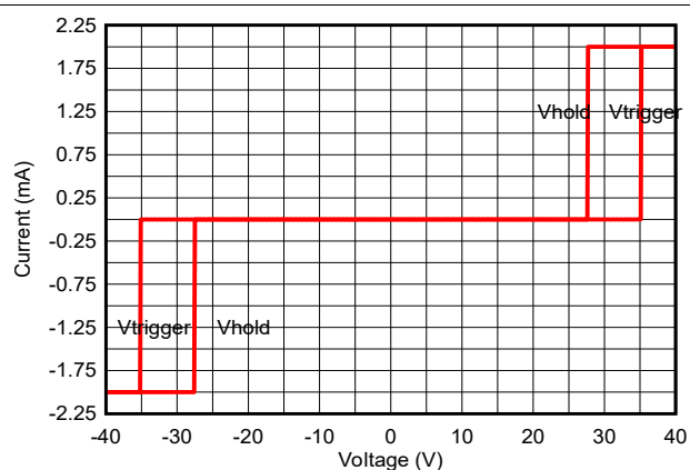
图 5-4. DC-IV 曲线
