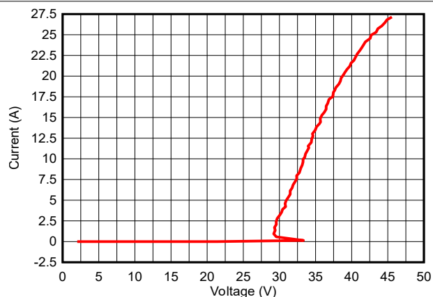
图 5-2. 负 TLP 曲线
