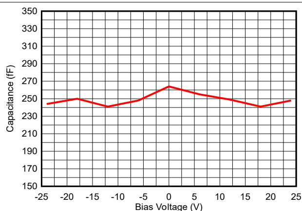
图 5-3. 偏置电压与电容间的关系
