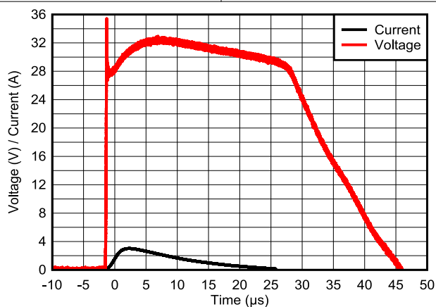
图 5-5. 8/20 \mu s 浪涌响应
