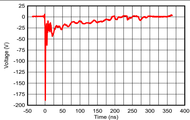
图 5-6. -8kV 钳位 IEC 波形
