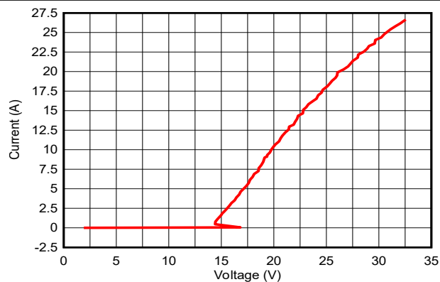
图 5-4. 负 TLP 曲线
