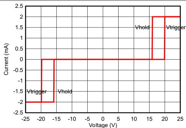
图 5-2. 直流 I-V 曲线
