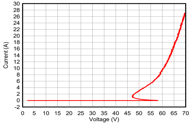
图 5-7. 正 TLP 曲线
