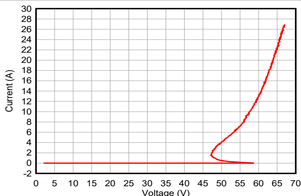
图 5-1. 正 TLP 曲线
