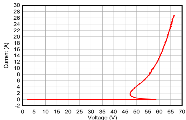
图 5-2. 负 TLP 曲线
