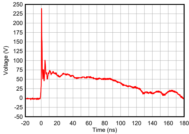
图 5-9. +8kV 钳位 IEC 波形
