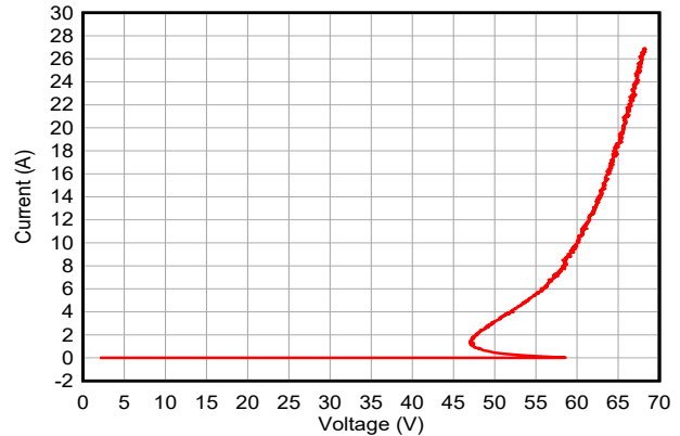
图 5-8. 负 TLP 曲线
