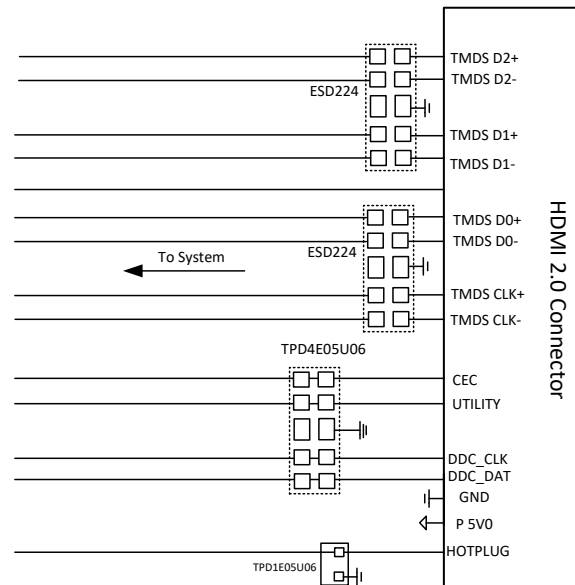
典型应用原理图
