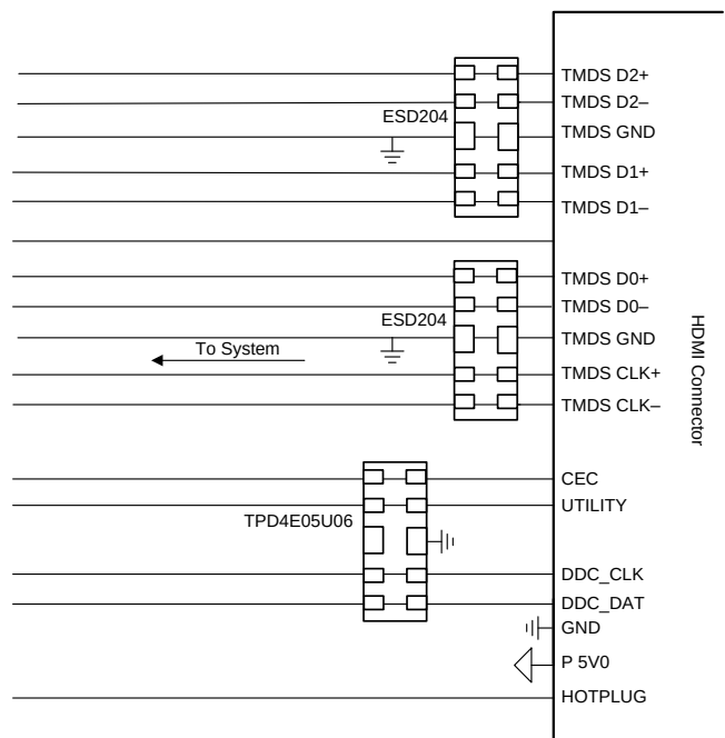
典型应用原理图
