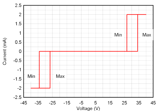
图 7-6. DC Voltage Sweep I-V Curve
