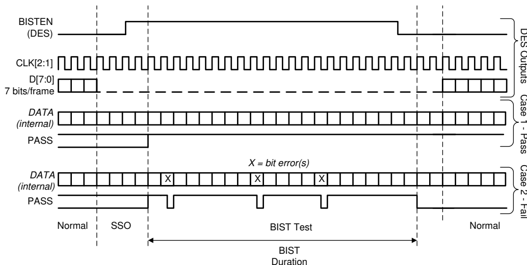
图 7-14. BIST Waveforms
