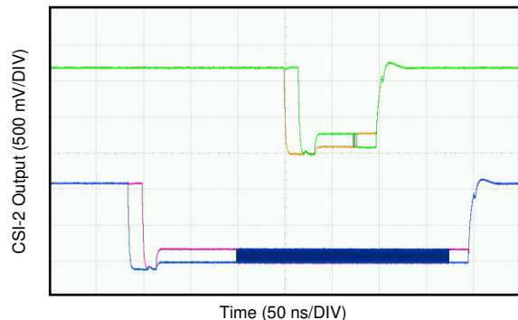
图 6-5. CSI-2 DATA and CLK Output
