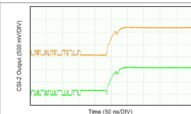
图 4-12. CSI-2 End of Transmission (EoT)
