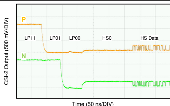
图 6-7. CSI-2 Start of Transmission (SoT)
