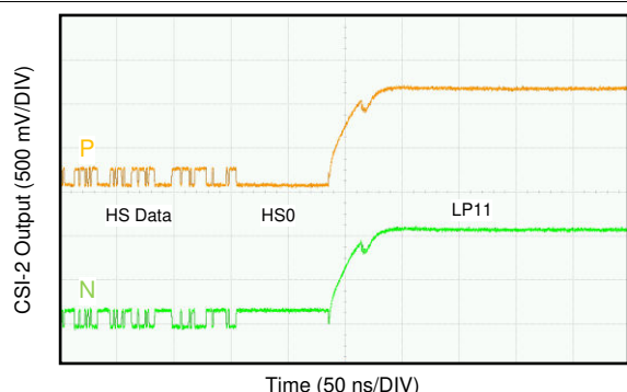
图 6-8. CSI-2 End of Transmission (EoT)
