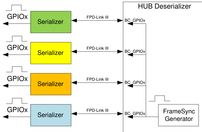
图 5-16. Internal FrameSync
