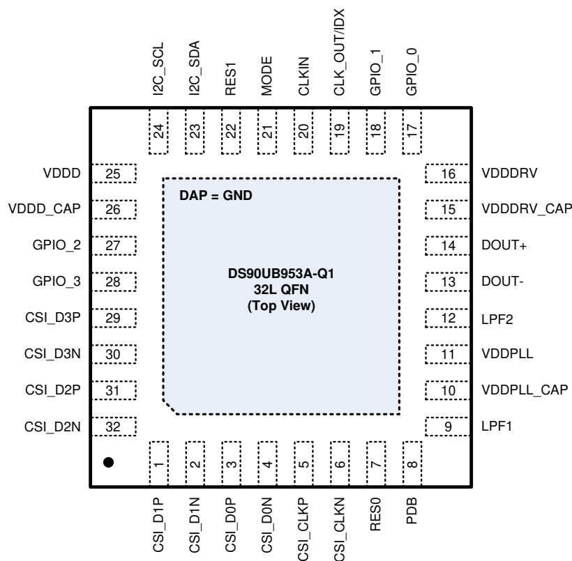
图 4-1. RHB 封装 32 引脚 VQFN 俯视图
