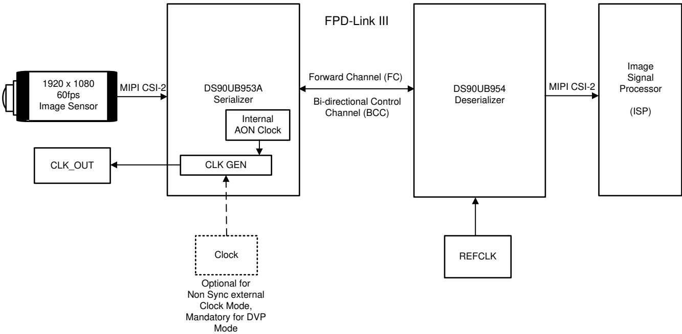
图 6-6. 时钟系统图
