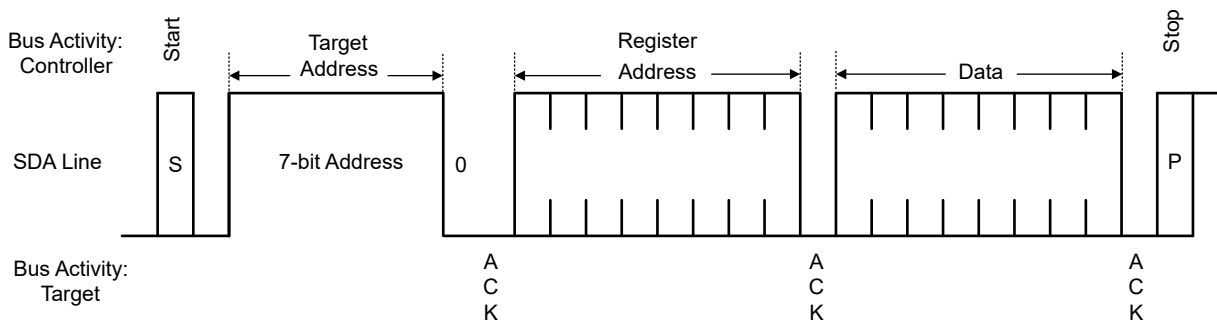
图 6-11. I2C 总线写入
