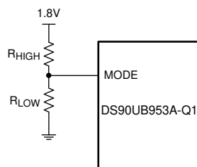
图 6-7. MODE 配置
