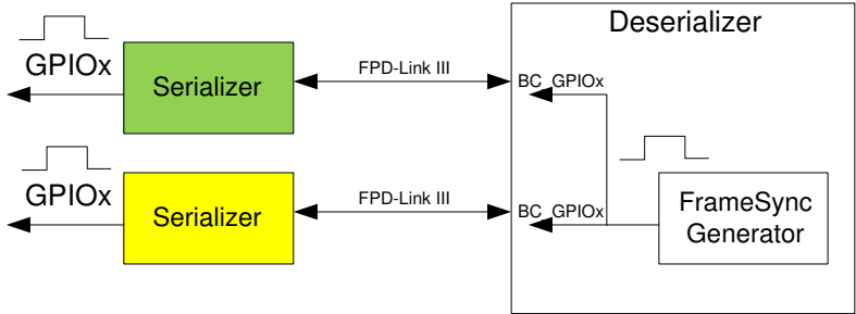
图 6-5. 内部帧同步
