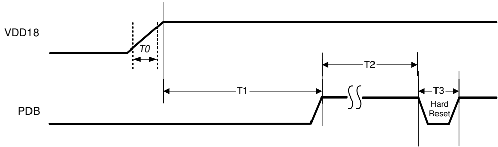
图 7-8. 电源时序
