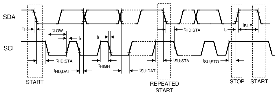
图 5-2. I²C 串行控制总线计时
