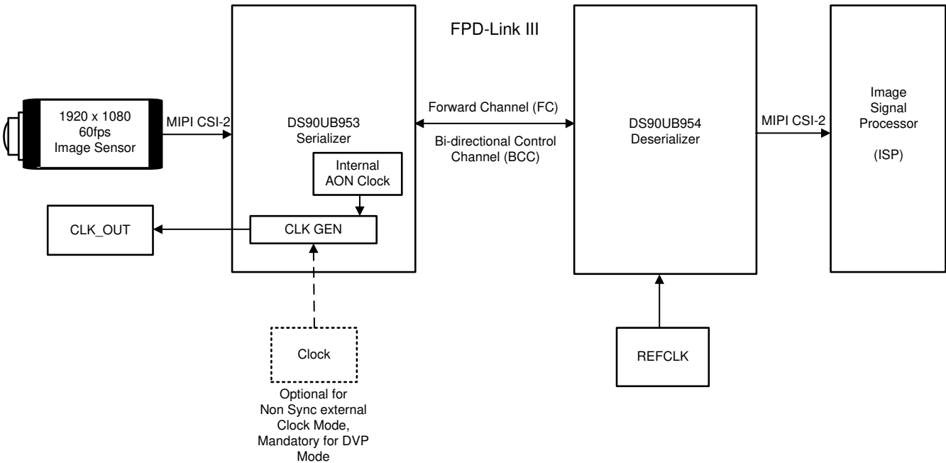
图 6-6. 时钟系统图
