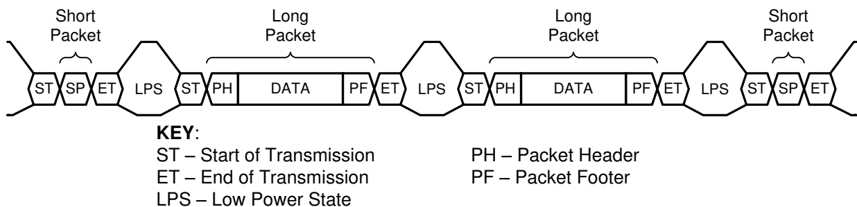
图 6-1. 包含短数据包和长数据包的 CSI-2 协议层
