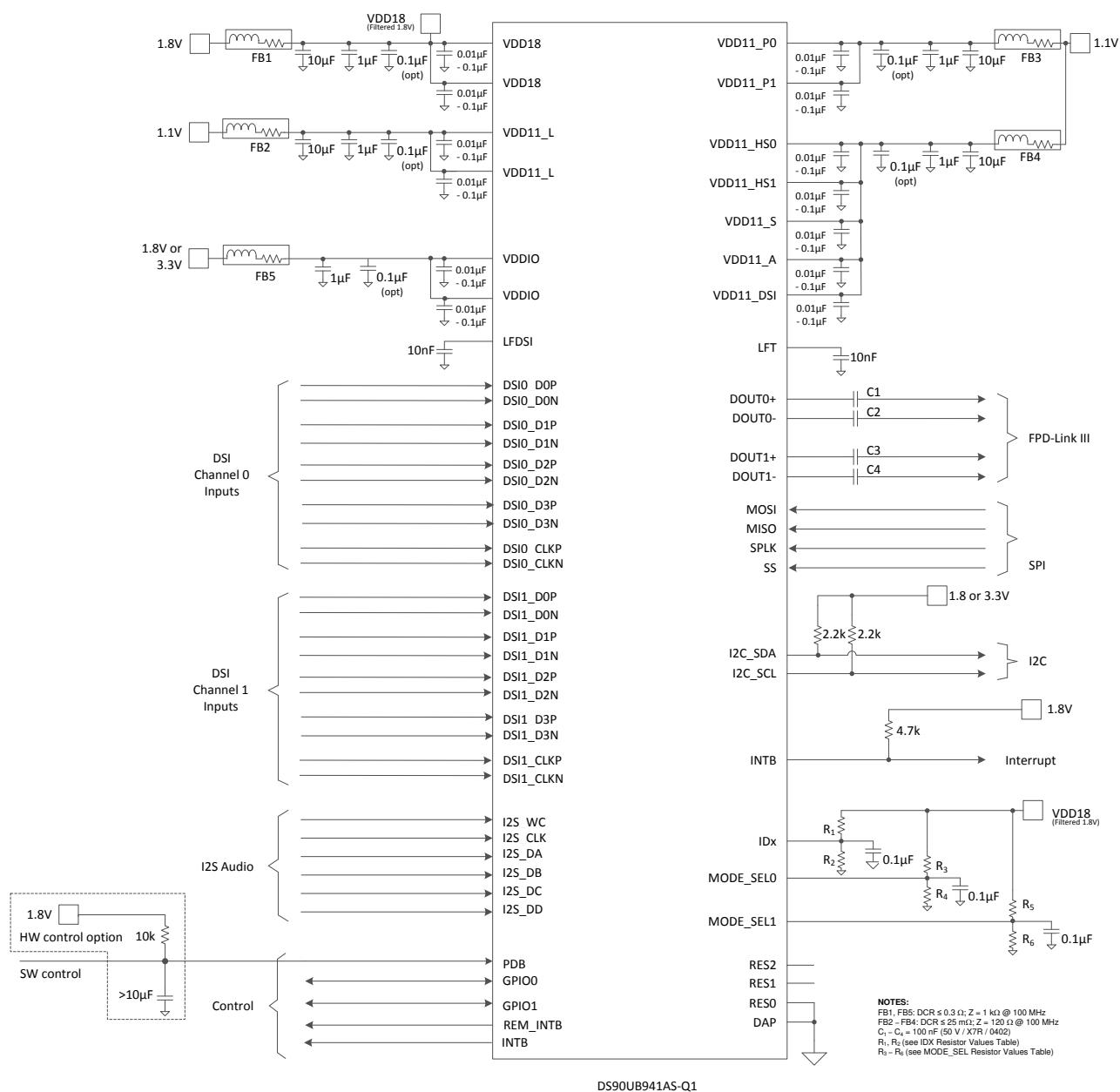
图 9-1. 典型连接图 - STP
