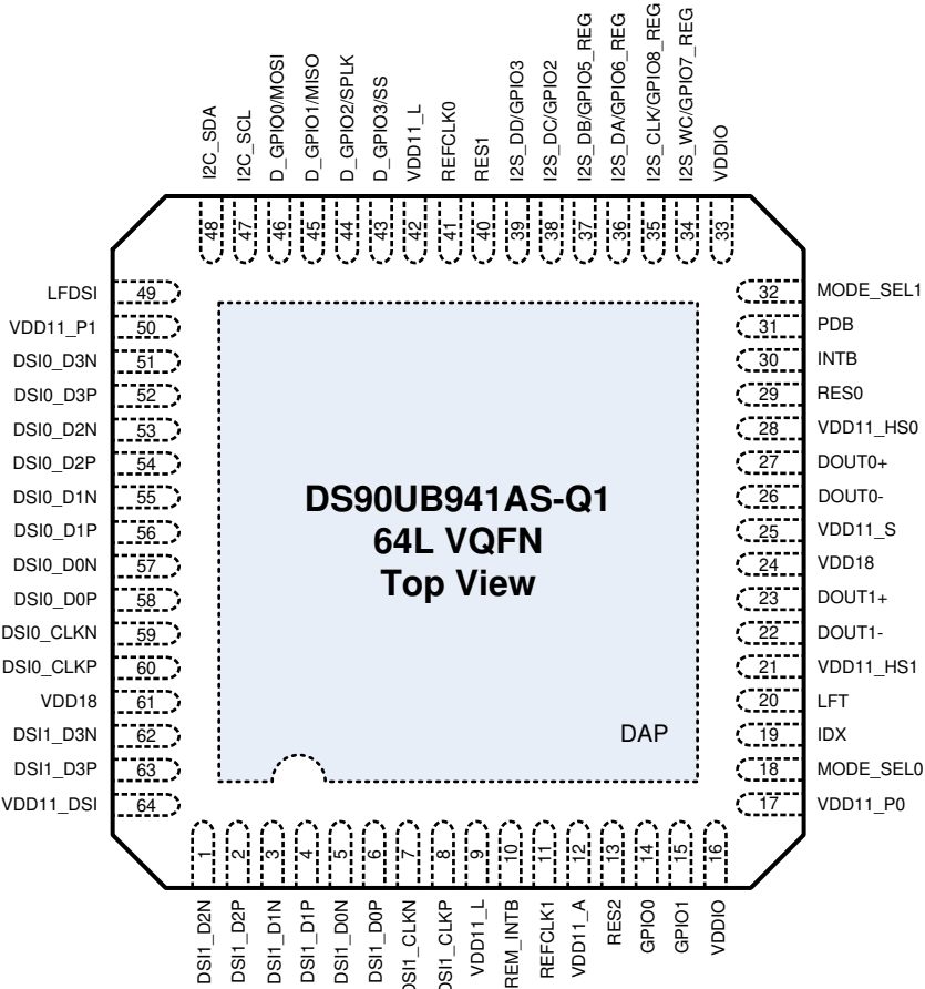
图 6-1. RTD 封装 64 引脚 VQFN 顶视图
