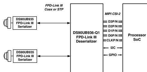
典型应用原理图
