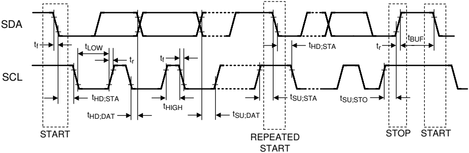
图 5-2. I 2 C 串行控制总线计时
