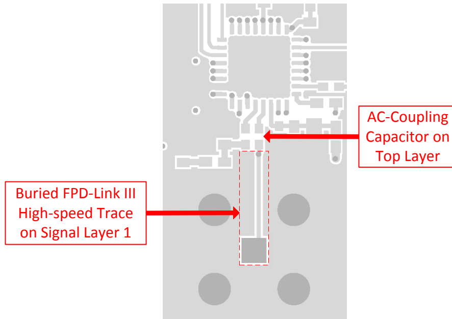
图 7-11. DS90UB935-Q1 串行器 DOUT+ 布线布局
