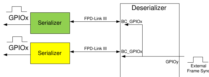
图 6-4. 外部帧同步
