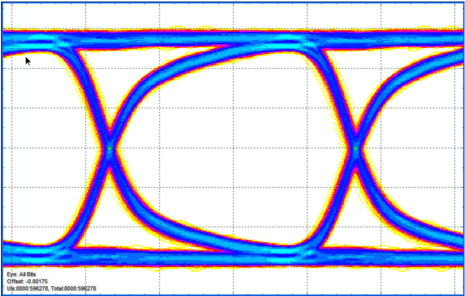
图 5-3. 来自串行器输出的 FPD-Link III 正向通道的眼图。垂直标度：100mV/DIV，水平标度：100ps/DIV
