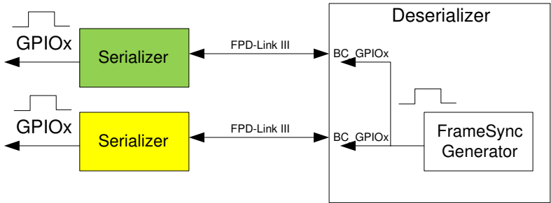
图 6-5. 内部帧同步
