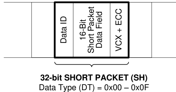
图 6-2. CSI-2 短数据包结构
