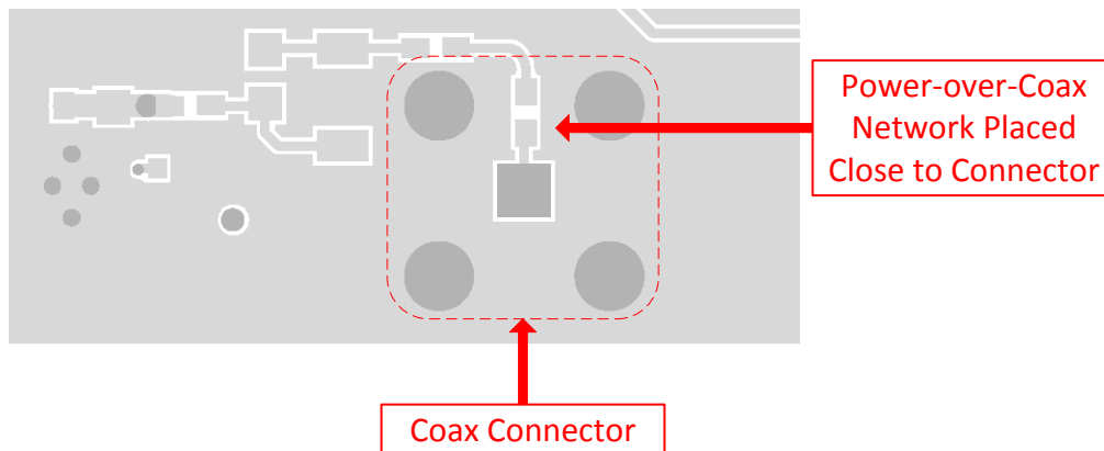
图 7-12. DS90UB935-Q1 同轴电缆供电布局
