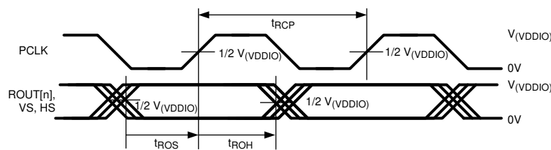
图 4-7. Deserializer Output Setup/Hold Times
