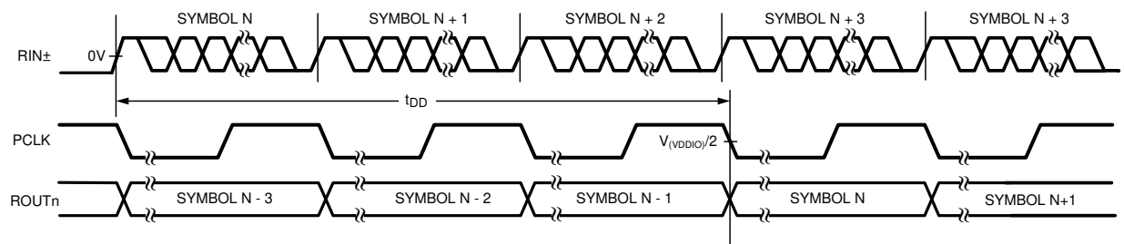
图 4-6. Deserializer Delay
