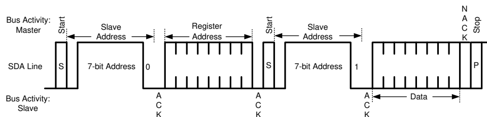
图 7-10. Read Byte
