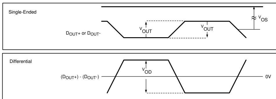
图 6-6. Serializer VOD Diagram
