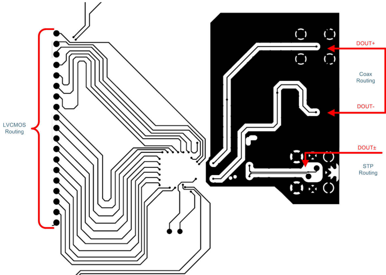
图 8-2. DS90UB913A-Q1 Serializer Example Layout
