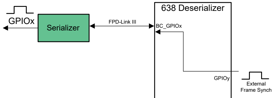
图 7-10. External FrameSync
