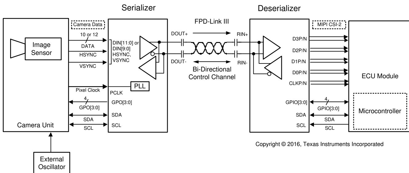
图 7-5. DS90UB633A-Q1/662-Q1 Operation in PCLK mode
